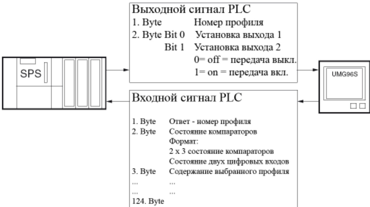
Диаграмма. Передача данных с PLC - UMG96S
