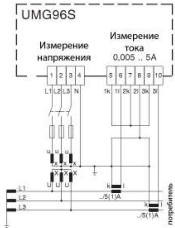
Схема: Пример подключения 6 3 трансформатора напряжения и 2 трансформатора тока.
