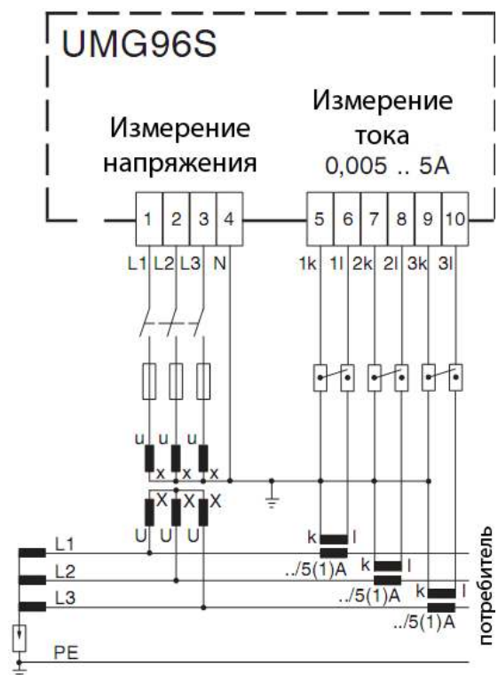
Схема: Пример подключения 8 Измерение в IT сетях с 3 трансформаторами напряжения и 3 трансформаторами тока.
