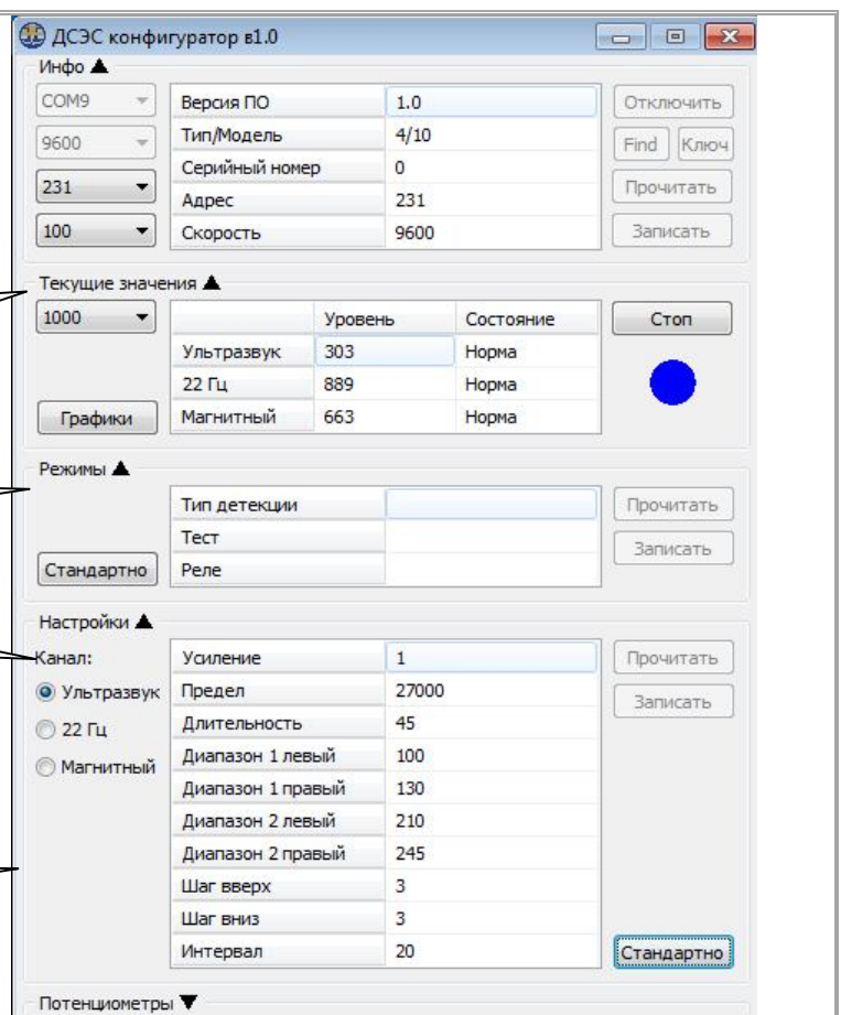
Рисунок 3. Интерфейс программы ДСЭС конфигуратор v1.0
