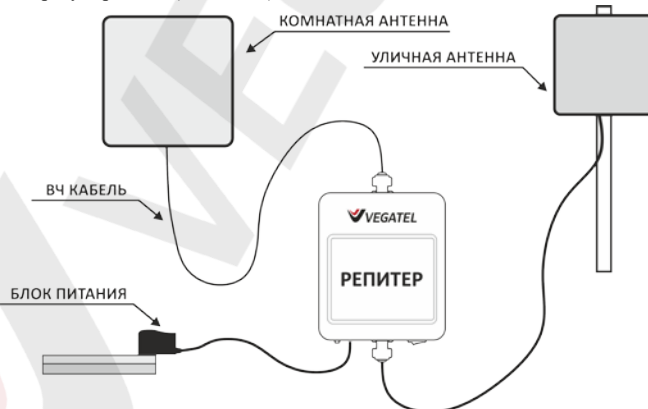
СХЕМА ПОДКЛЮЧЕНИЯ РЕПИТЕРА
