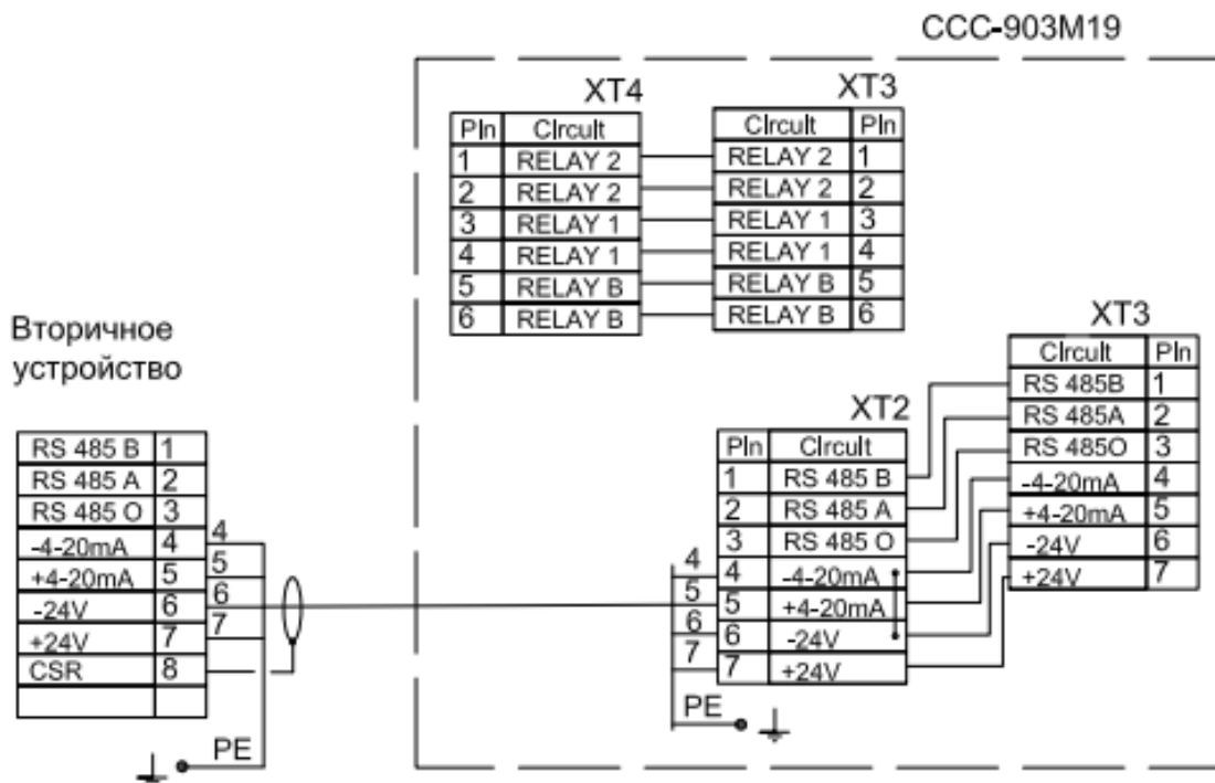
Рис.1 Схема подключения CCC-903M19 к вторичным устройствам по аналоговому выходу 4-20мА
