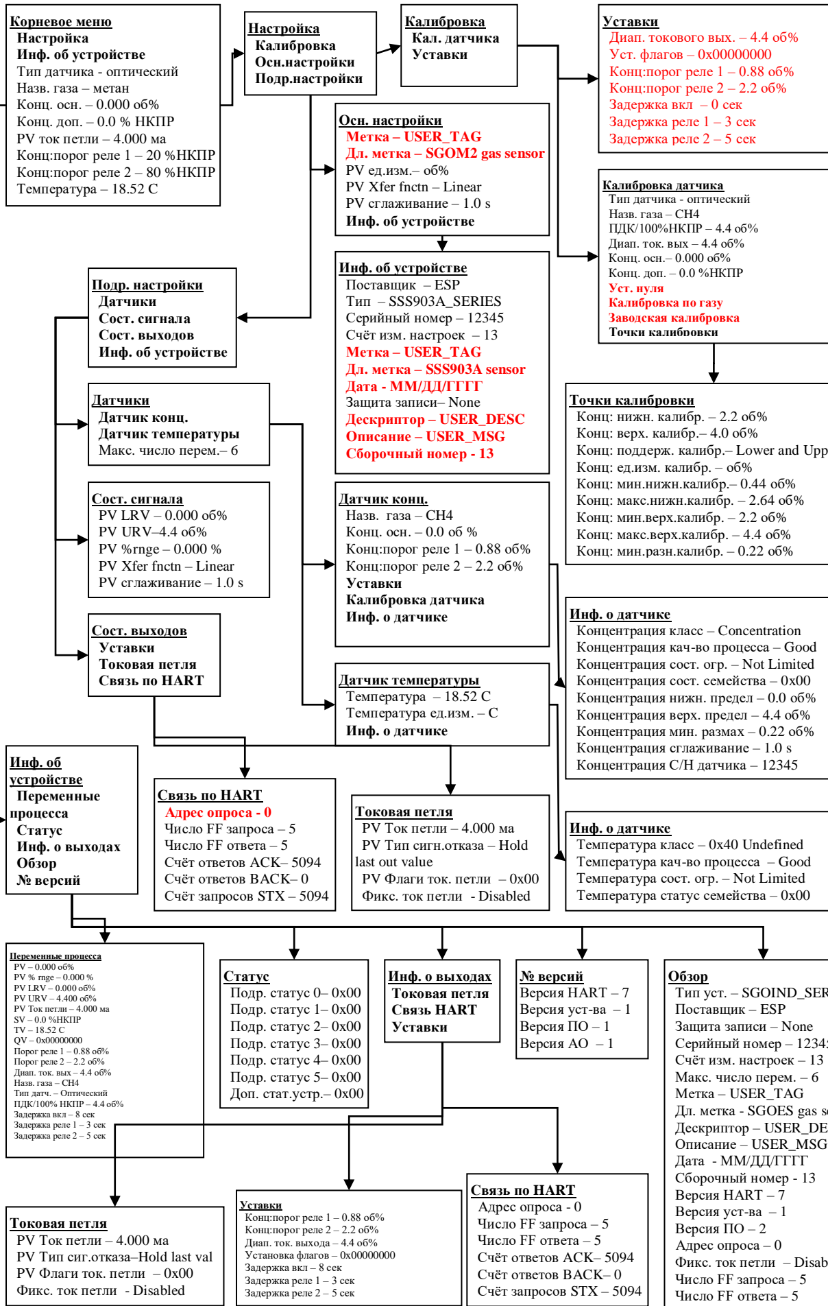
Рисунок 11 - Структура русскоязычного HART меню
