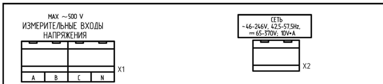
Рисунок Б.7 – Расположение элементов измерительного клеммного отсека приборов «Ресурс-ПКЭ-1.Х-оэ-Х»
