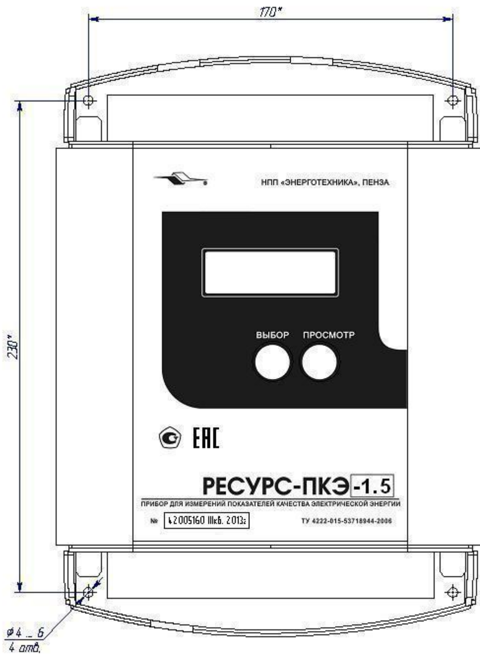
Рисунок А.3 – Установочные размеры «Ресурс-ПКЭ-Х.Х-оХ-Х»
