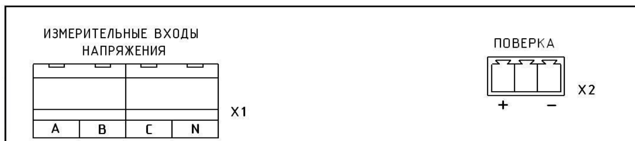
Рисунок Б.5 – Расположение элементов измерительного клеммного отсека приборов «Ресурс-ПКЭ-1.Х-ои-Х»
