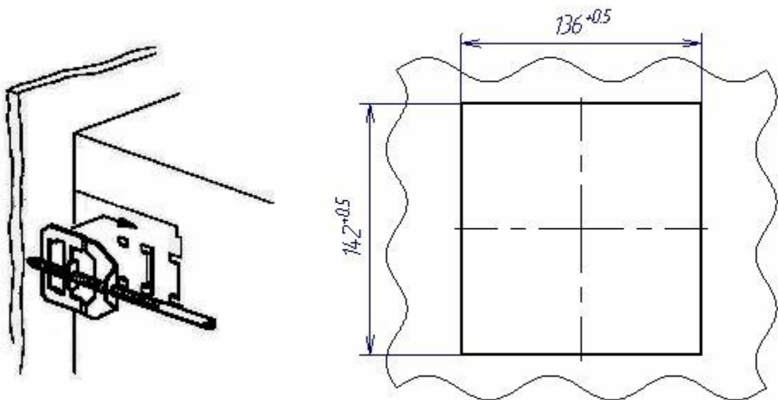
Схема крепления
