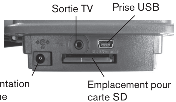
Fig. 1: Connexions
