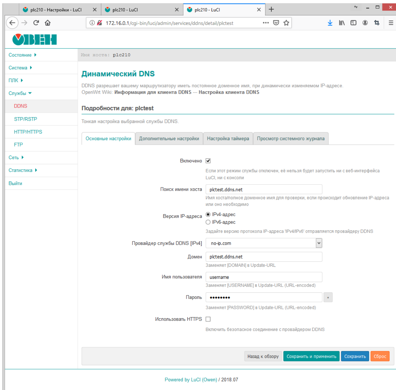
Рисунок 6-5: Страница редактирования DDNS записи
