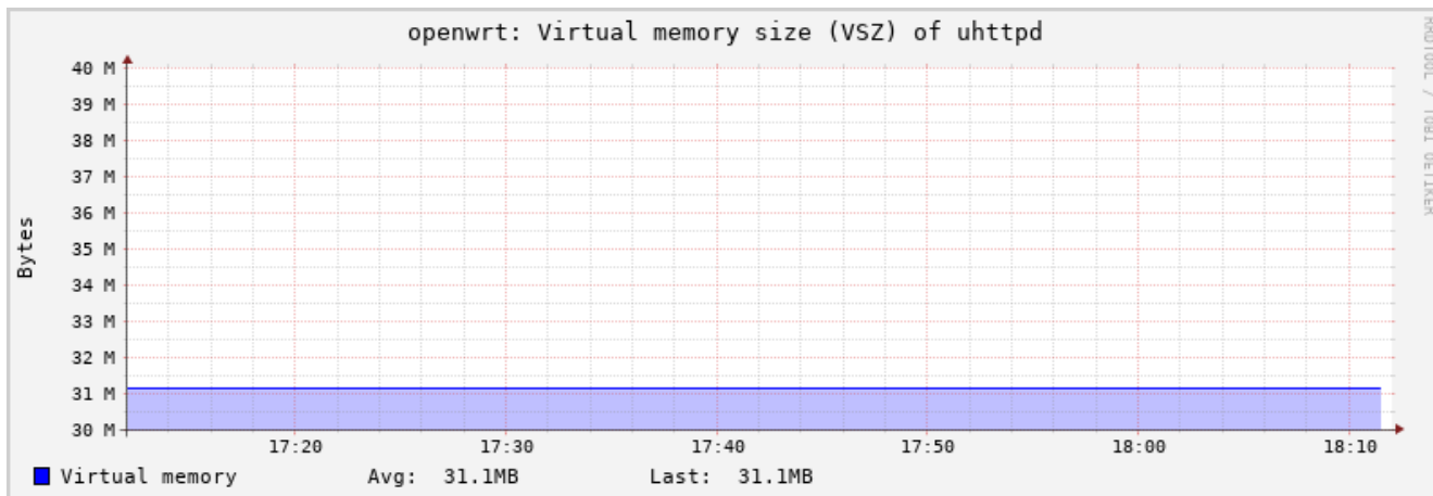
Рисунок 8-12: Статистика. График VSZ процесса
