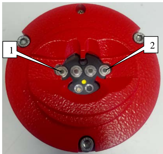
Рисунок 2 – Лицевая часть ИПЭС-IR4000
