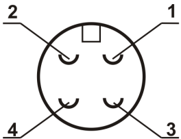
Разъем PC4 (розетка) со стороны монтажа
