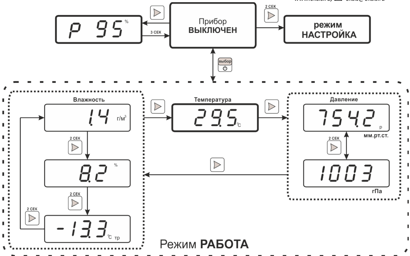
Рисунок 5.14 Режим РАБОТА ИВТМ-7 М 1(-Д)
