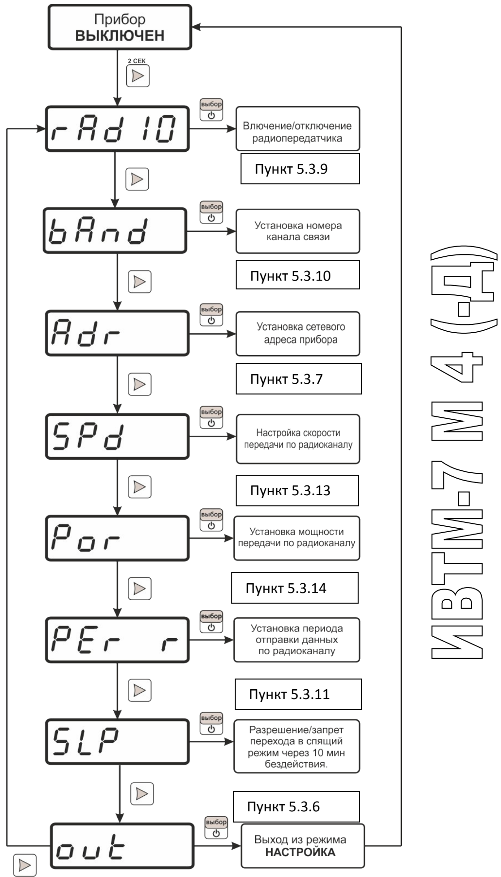
Рисунок 5.21 Схема режима НАСТРОЙКА ИВТМ-7 М 4(-Д)
