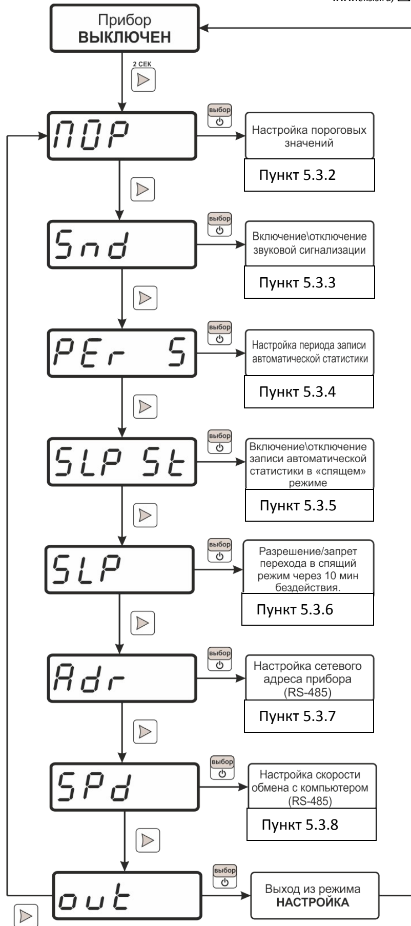
Рисунок 5.20 Схема режима НАСТРОЙКА ИВТМ-7 М 3(-Д)
