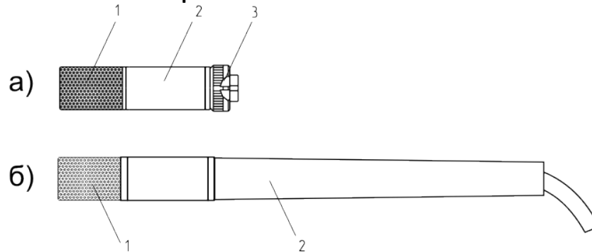
Рисунок 3.12 Измерительные преобразователи
