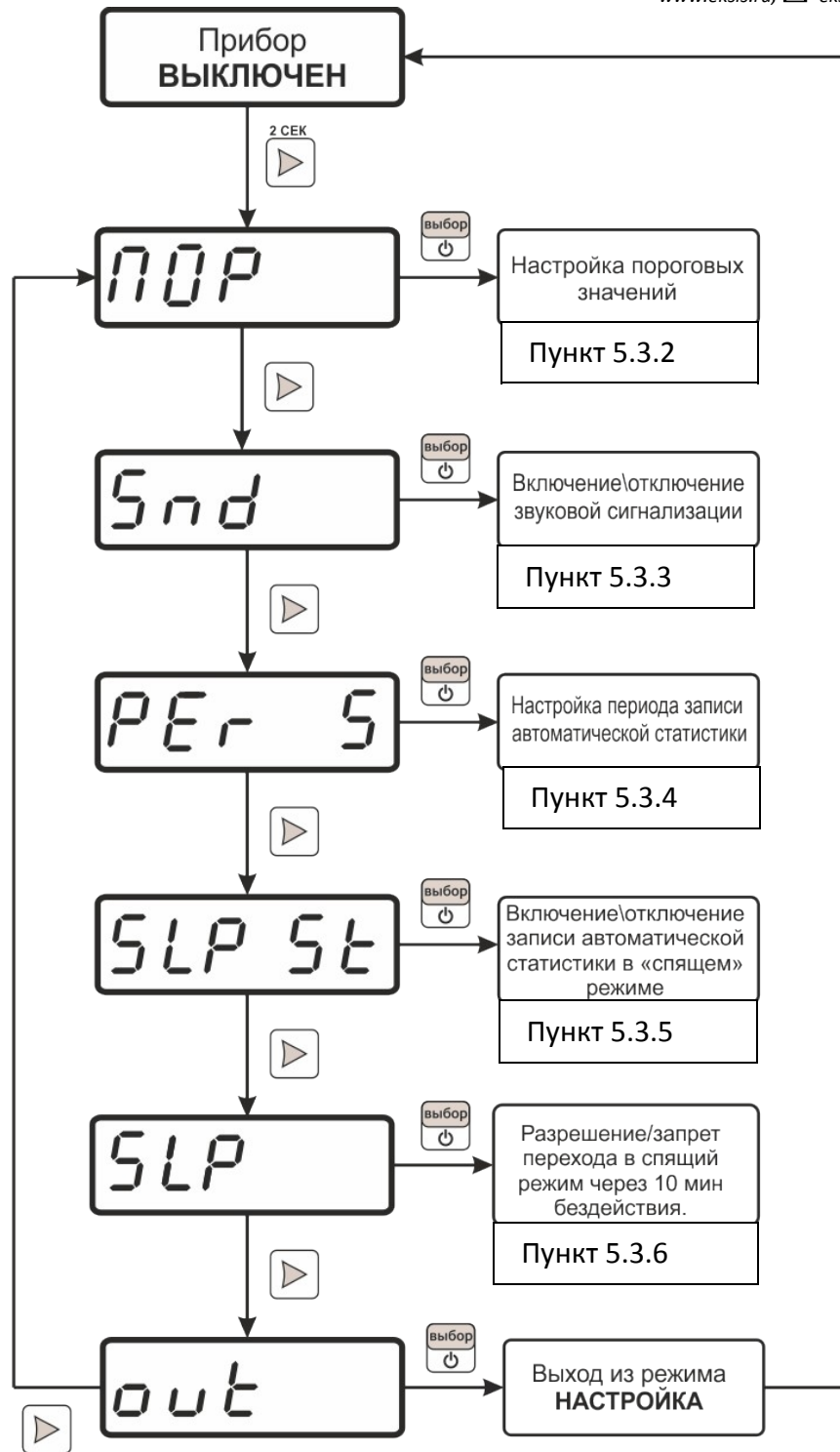
Рисунок 5.22 Схема режима НАСТРОЙКА ИВТМ-7 М 6(-Д)
