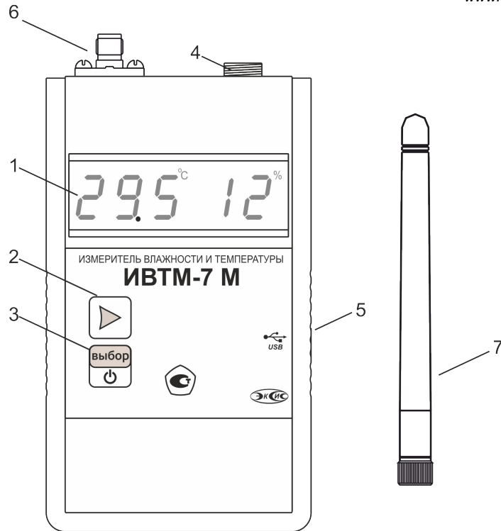
Рисунок 3.4 Внешний вид измерительного блока ИВТМ-7 М 4(-Д)
