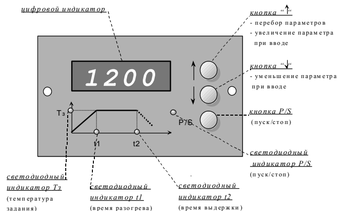
Рис. 3.2. Лицевая панель регулятора.
