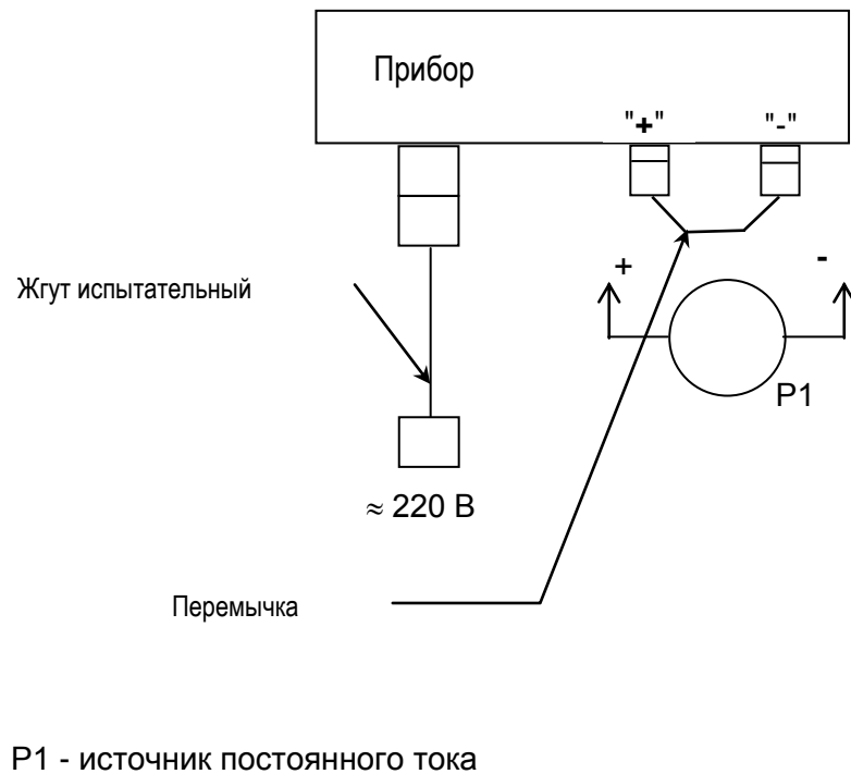
Рисунок 8.1 - Схема проверки прибора.
