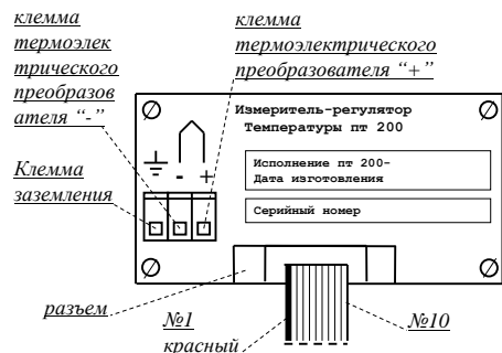
Рисунок 3.3 - Задняя панель прибора
