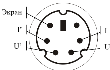
MiniDin 6, вид со стороны пайки
