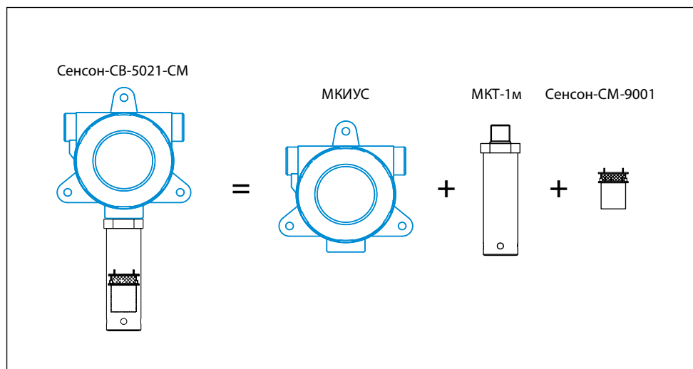
Рис.А4. Система газоаналитическая "Сенсон-СВ-5021-СМ"
