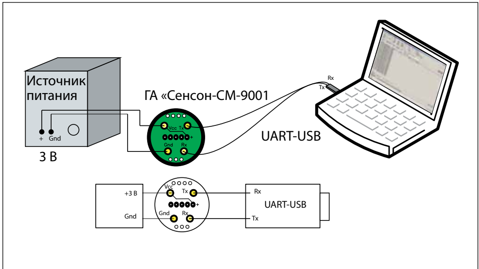
Рис.3. Общая схема подключения газоанализатора "Сенсон-СМ-9001"
