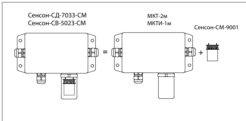
Рис.А3. Система газоаналитическая "Сенсон-СД-7033-СМ" и "Сенсон-СВ-5023-СМ"
