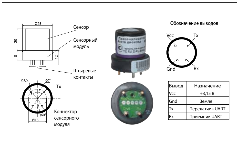
Рис.2. Габаритный чертеж, расположение и назначение выводов газоанализатора "Сенсон-СМ-9001"
