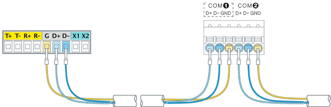
Рис. 40 –Подключение проводов шины MTBus к контроллерам TRIM5 модификаций XXXX-20-2
