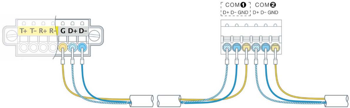
Рис. 39 –Подключение проводов шины MTBus к контроллеру TRIM5-3012-65-2
