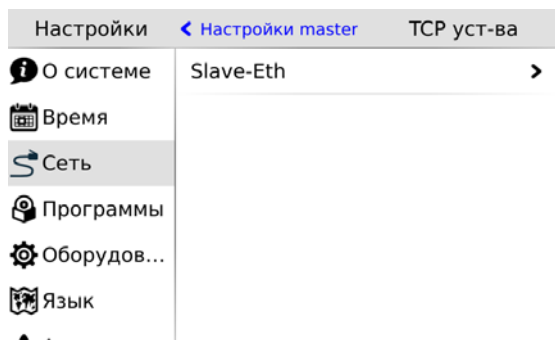
Рис. 59 – slave-устройства Modbus
