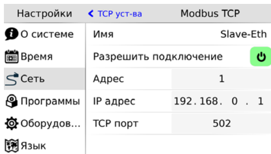
Рис. 60 – Настройка Modbus TCP slave
