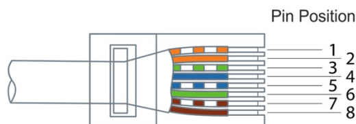
Рис. 36 - Цоколёвка RJ-45
