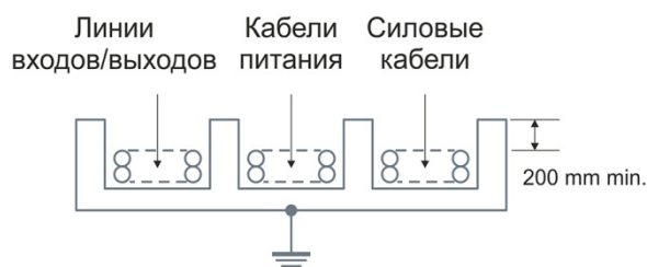
Рис. 26 - Горизонтальные каналы
