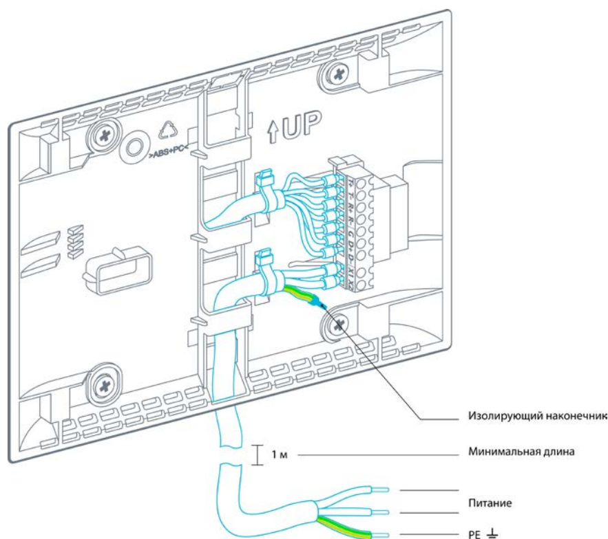
Рис. 29 – Подключение сенсорной панели к питающей сети
