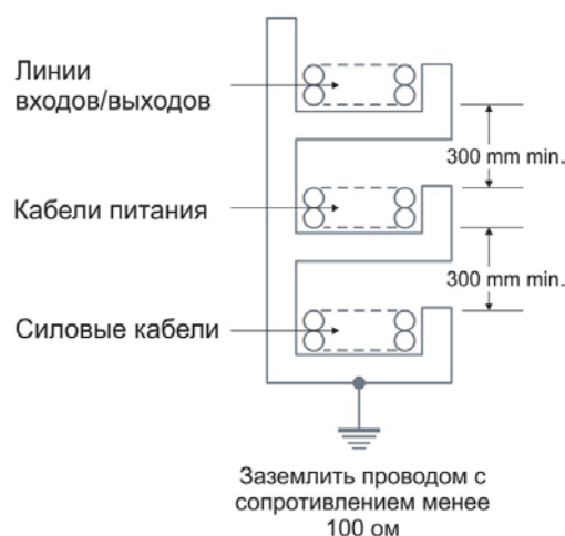
Рис. 25 - Подвесные каналы
