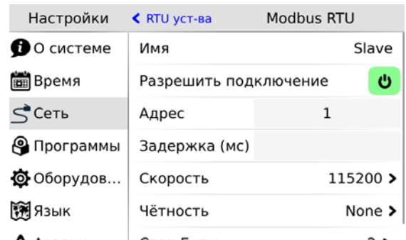
Рис. 61 – Настройка Modbus RTU slave
