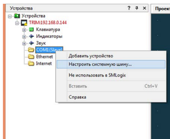
Рис. 37 – Конфигурирование режима работы COM1
