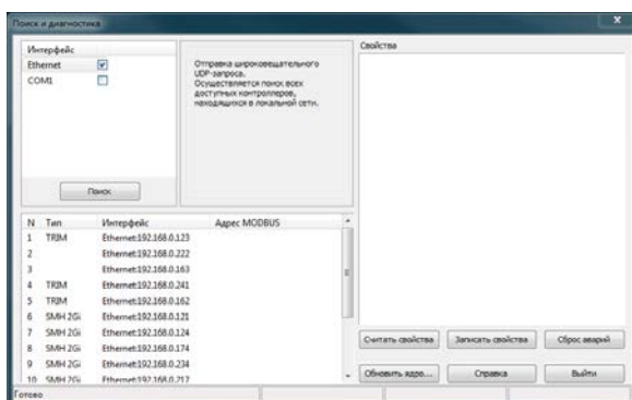
Рис. 82 – Поиск и диагностика
