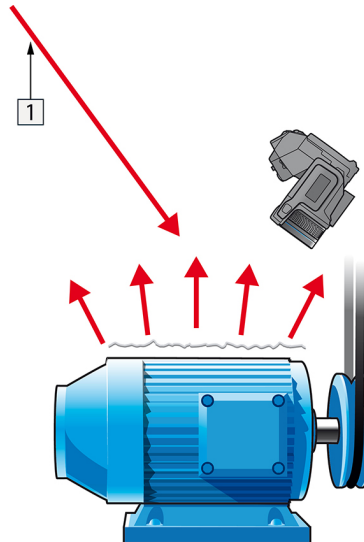
Рисунок 33.5 Измерение видимой температуры от алюминиевой фольги.
