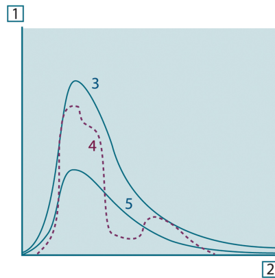
Рисунок 36.8 Спектральная излучательная способность трех типов излучателей 1: Спектральная излучательная способность; 2: Длина волны; 3: Черное тело; 4: Избирательный излучатель; 5: Серое тело.
