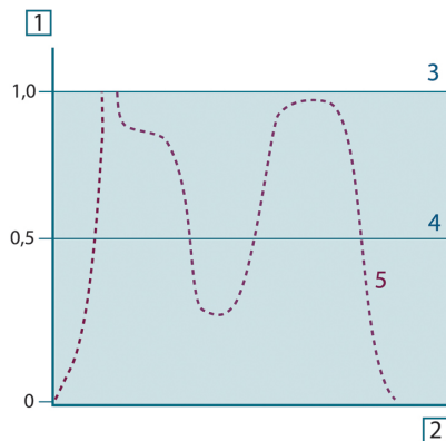
Рисунок 36.9 Спектральный коэффициент излучения трех типов излучателей 1: Спектральный коэффициент излучения; 2: Длина волны; 3: Черное тело; 4: Серое тело; 5: Избирательный излучатель.
