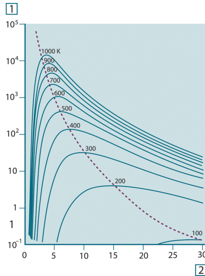
Рисунок 36.6 Кривые Планка, построенные в полулогарифмическом масштабе от 100 К до 1000 К. Пунктирная линия представляет геометрическое место точек максимума излучательной способности при каждой температуре согласно закону смещения Вина 1: Спектральная излучательная способность (Вт/см 2 (мкм)); 2: Длина волны (мкм).
