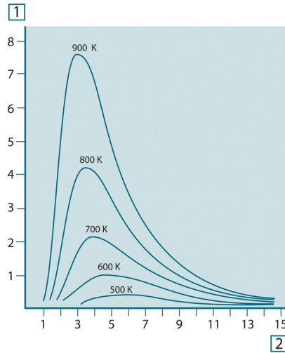
Рисунок 36.4 Кривые спектральной излучательной способности черного тела в соответствии с законом Планка, построенные для разных значений абсолютной температуры 1: Спектральная излучательная способность ( \text{Вт/см}^2 \times 10^3(\text{мкм}) ); 2: Длина волны (мкм).
