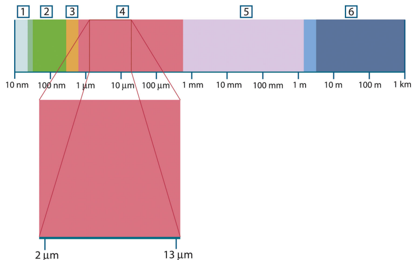
Рисунок 36.1 Спектр электромагнитного излучения 1: Рентген. лучи; 2: УФ; 3: Видимый; 4: ИК; 5: Микроволны; 6: Радиоволны.
