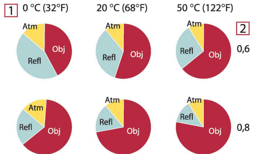
Рисунок 37.3 Относительные величины источников излучения при различных условиях измерений (LW-камера). 1: Температура объекта; 2: Светимость; Obj: Излучение объекта; Refl: Отраженное излучение; Atm: излучение атмосферы. Фиксированные параметры: \tau = 0,88 ; T_{\text{refl}} = 20^{\circ}\text{C} ; T_{\text{atm}} = 20^{\circ}\text{C} .
