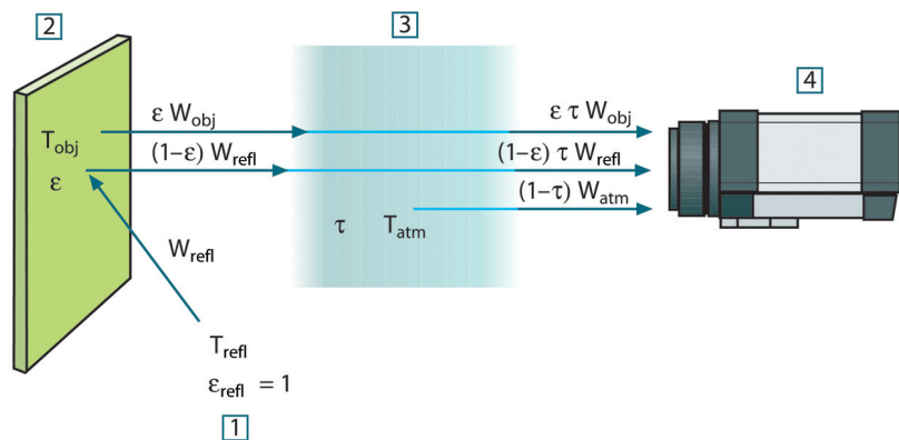
Рисунок 37.1 Схематическое представление ситуации при общих термографических измерениях 1: Среда; 2: Объект; 3: Атмосфера; 4: Камера
