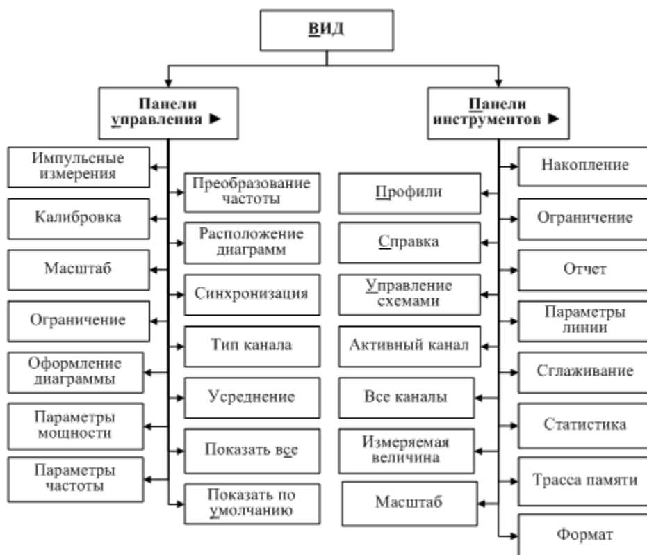
Рисунок 3.20 – Структура подменю «Вид»
