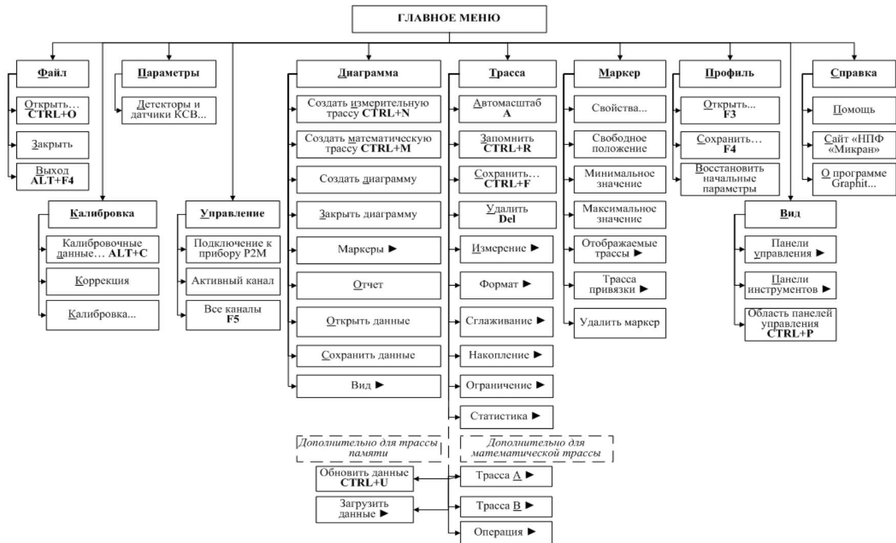
Рисунок 3.17 – Структура главного меню
