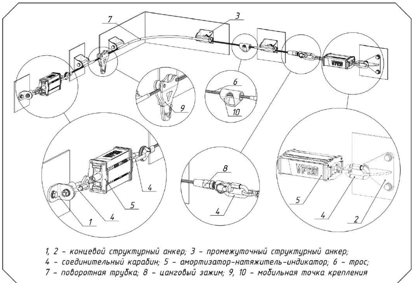
Рис.1 Основные составляющие анкерной линии «ТРОСЛАЙН»
