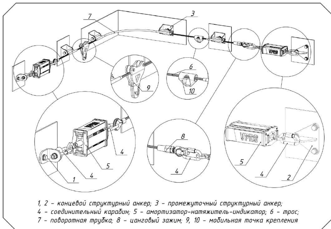
Рис. 2 Монтаж анкерной линии
