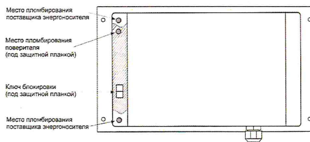
б) исполнение для щитового монтажа (вид сзади)
