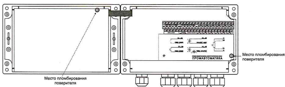
а) Места пломбирования (Вариант 1)
