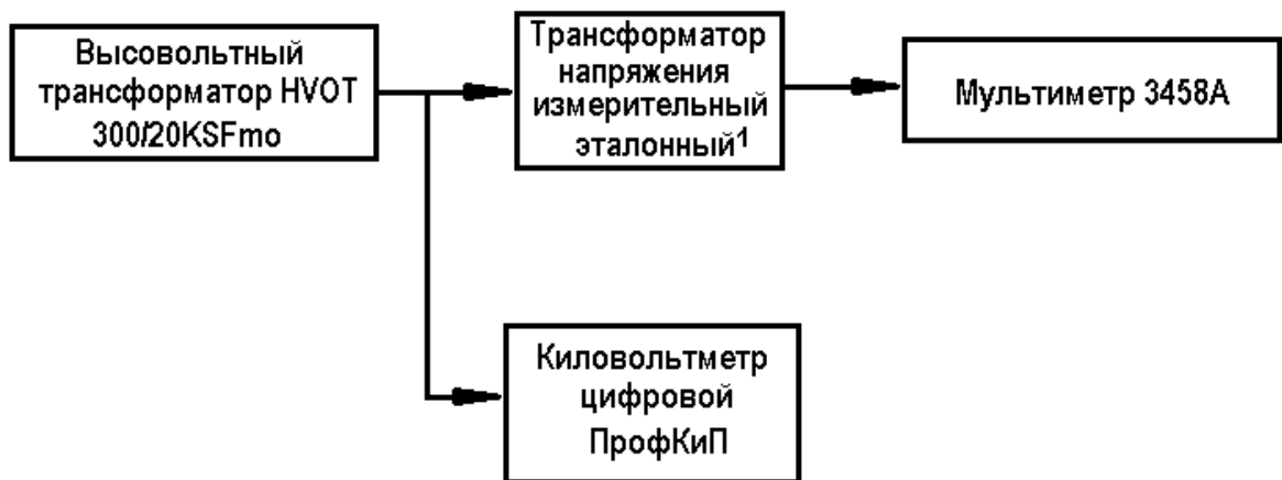
Рисунок 1-Структурная схема подключения приборов для определения относительной погрешности измерения среднеквадратических значений напряжения переменного тока синусоидальной формы частотой 50 Гц.
