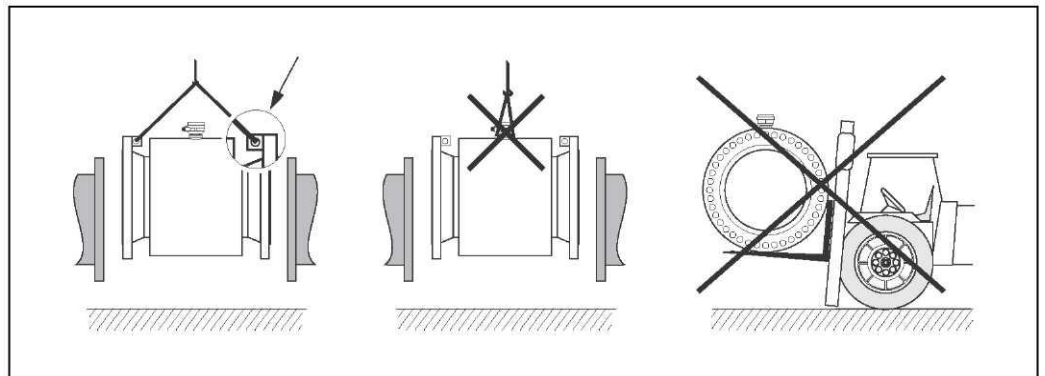
Рис. 5. Транспортировка сенсоров с ДУ > 300
