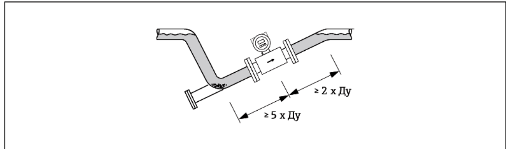
Рис. 8. Монтаж в частично заполненной трубе
