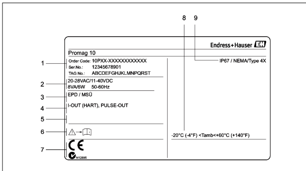
Рис. 1. Информация на заводской табличке трансмиттера Promag 10 (пример) :
