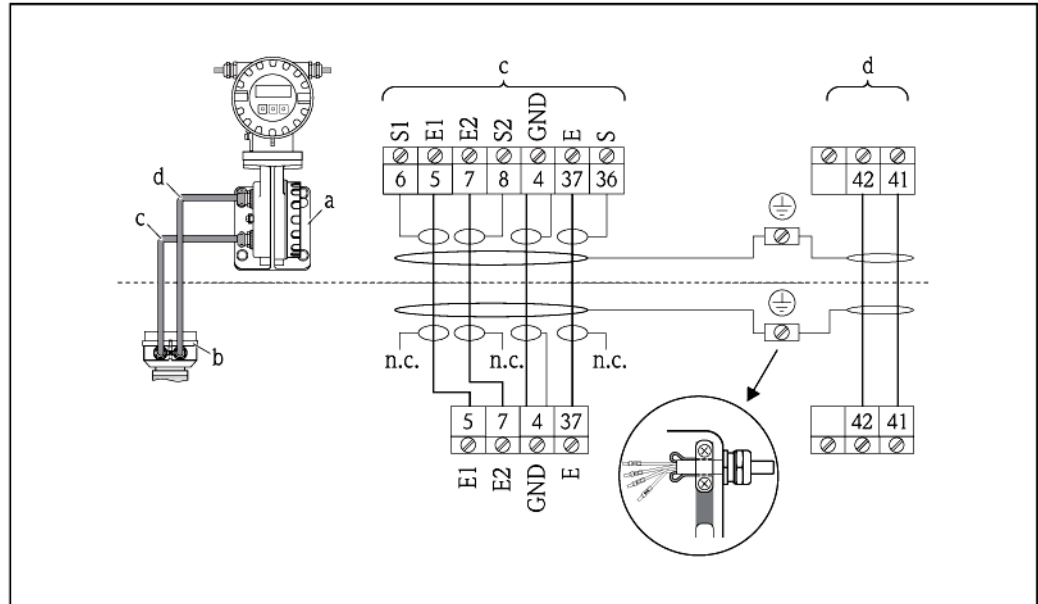
Рис. 28. Подключение приборов Promag H в отдельном исполнении
