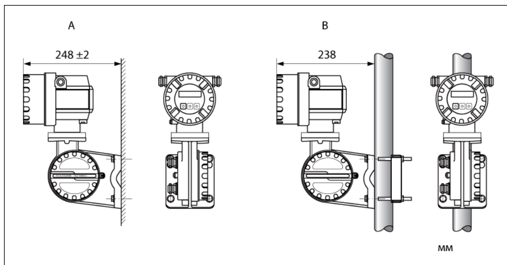
Рис. 25. Монтаж трансмиттера (раздельное исполнение)
