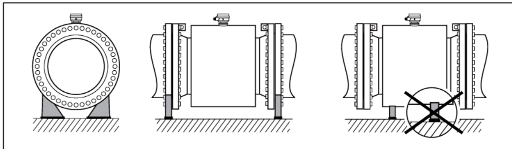
Рис. 14. Правильная организация опоры для больших номинальных диаметров ( D \geq 350 )
