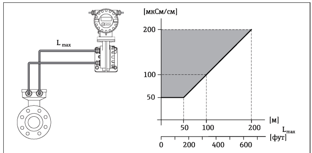
Рис. 16. Допустимая длина кабеля для раздельного исполнения
