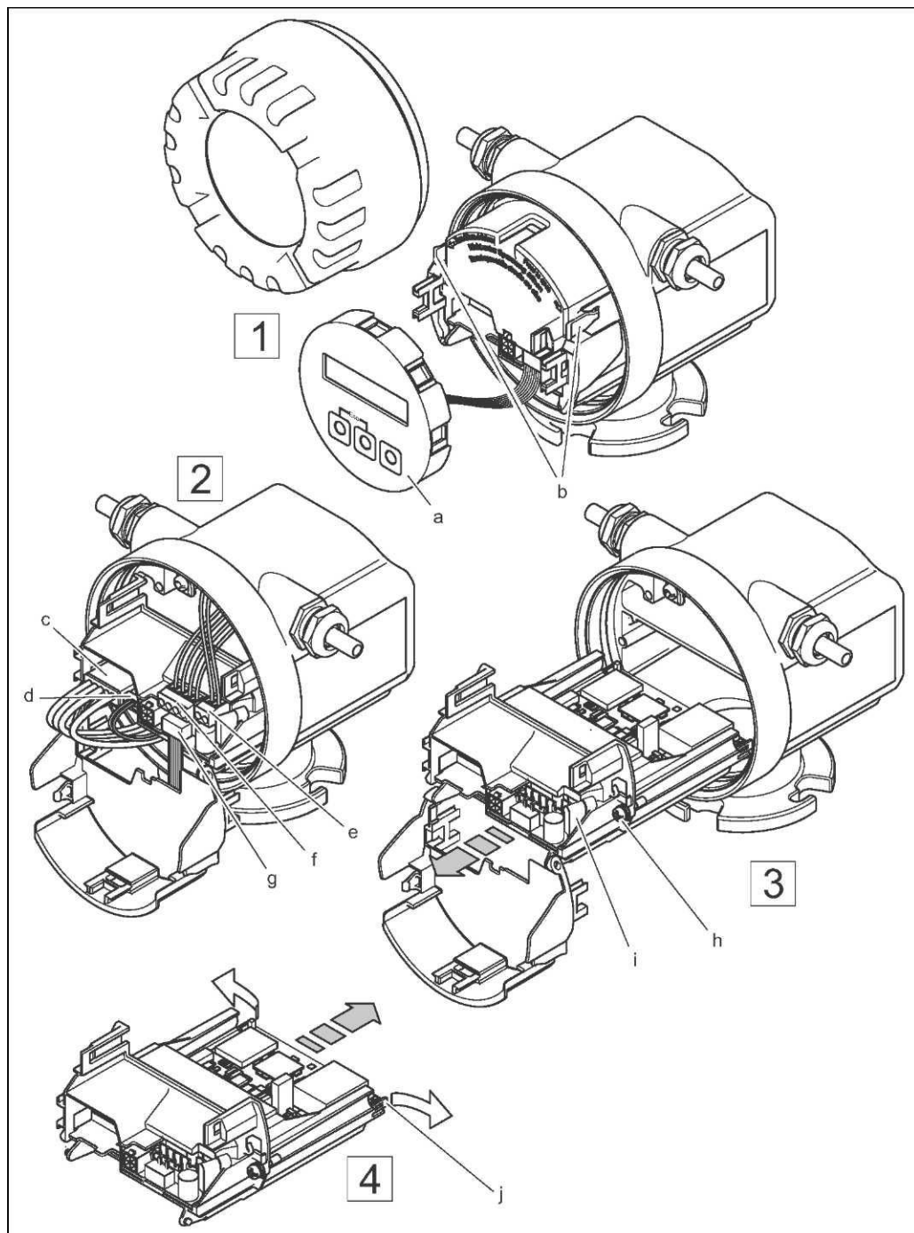
Рис. 46. Полевой корпус: установка и удаление печатных плат
