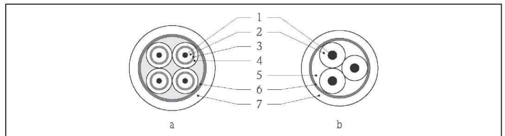
Рис. 29. Поперечное сечение кабеля
