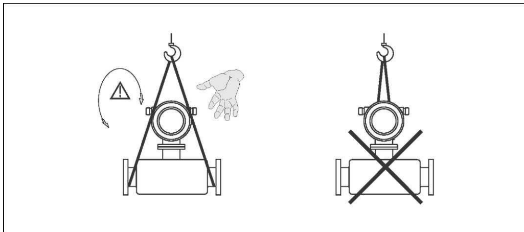
Рис. 4. Транспортировка сенсоров с DN \leq 300
