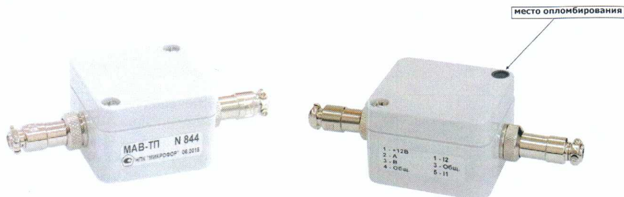
Рисунок 2 - Общий вид модуля с местом пломбировки от несанкционированного доступа
