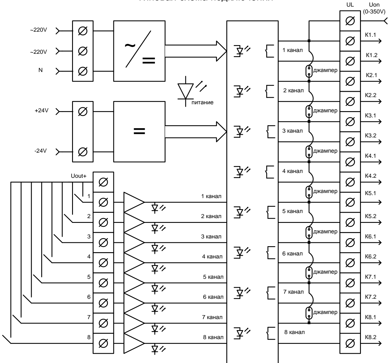
Типовая схема подключения
