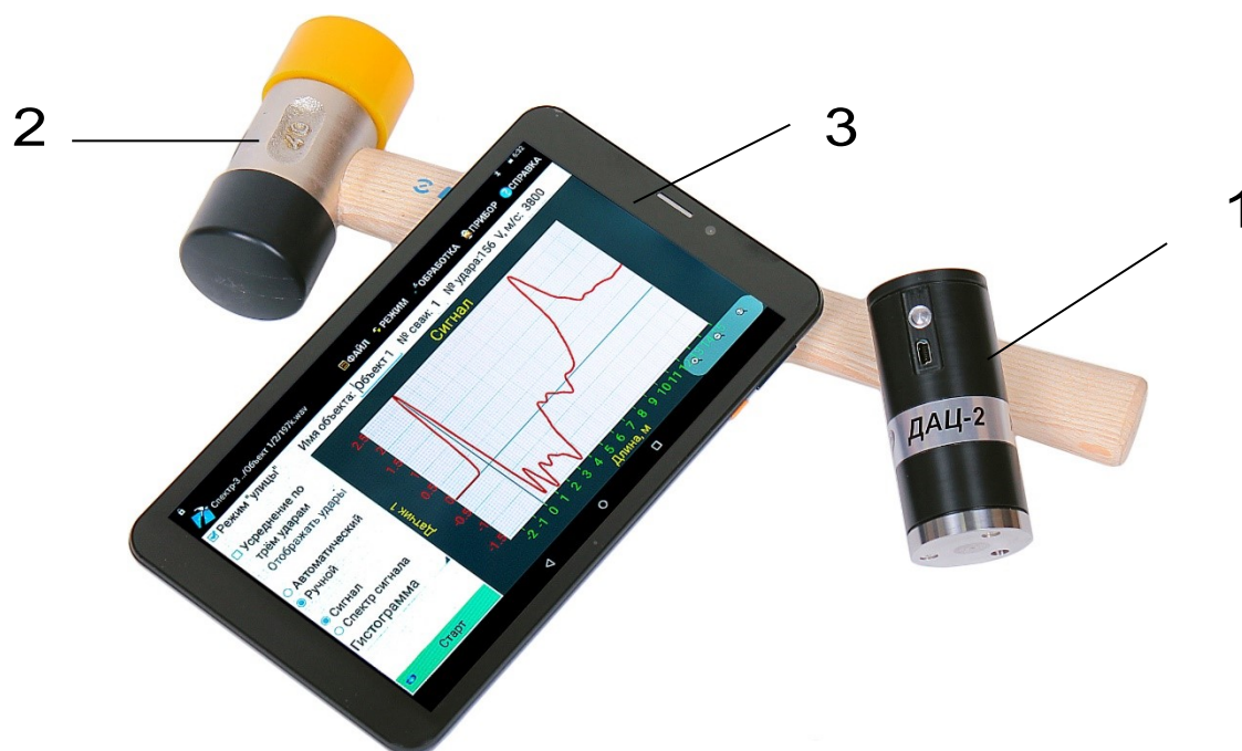
Рисунок 3.1 - Общий вид прибора Спектр-4.31.
