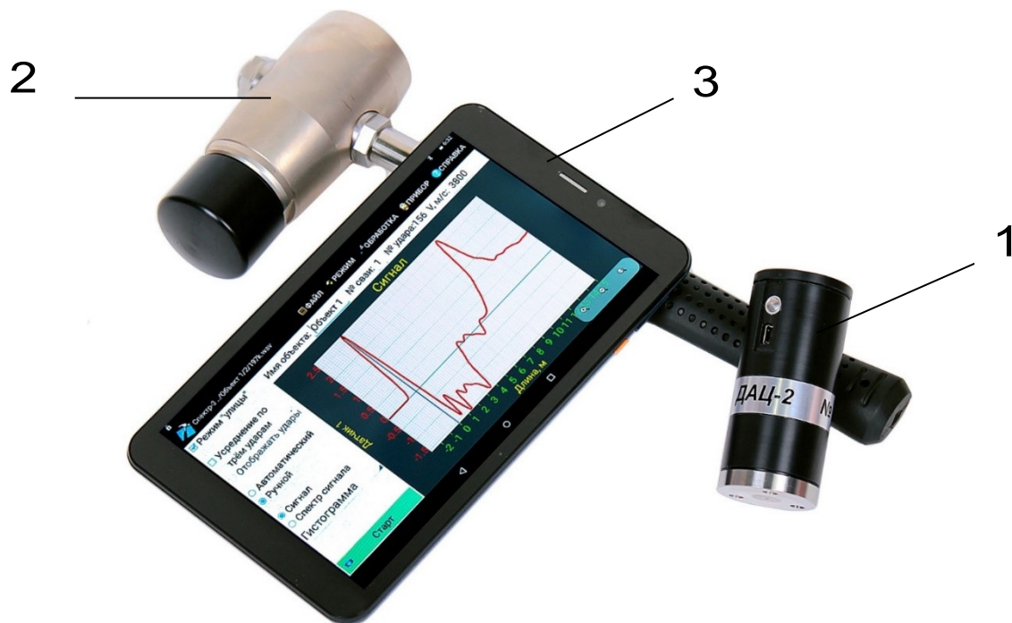
Рисунок 3.2 - Общий вид прибора Спектр-4.32.
