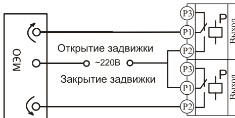
Подключение электродвигателя
