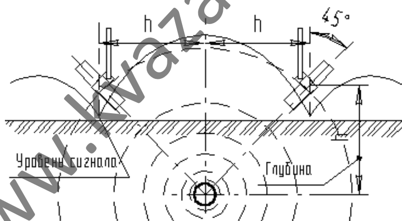
Рис.7.3. Определение глубины методом 45^\circ .
