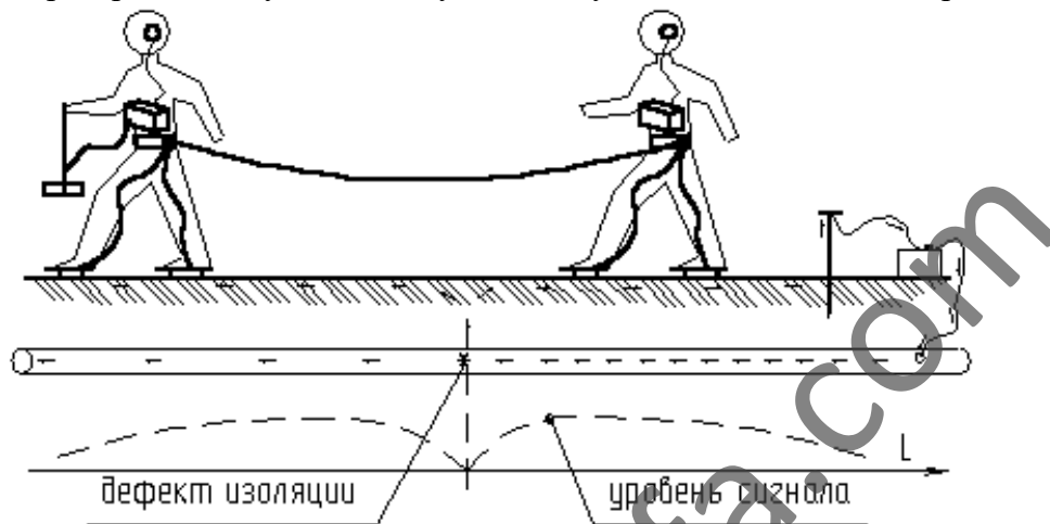
Рис.7.4. Схема определения местоположения дефекта изоляции.
