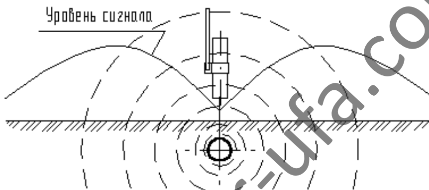
Рис.7.2. Поиск по минимуму сигнала.
