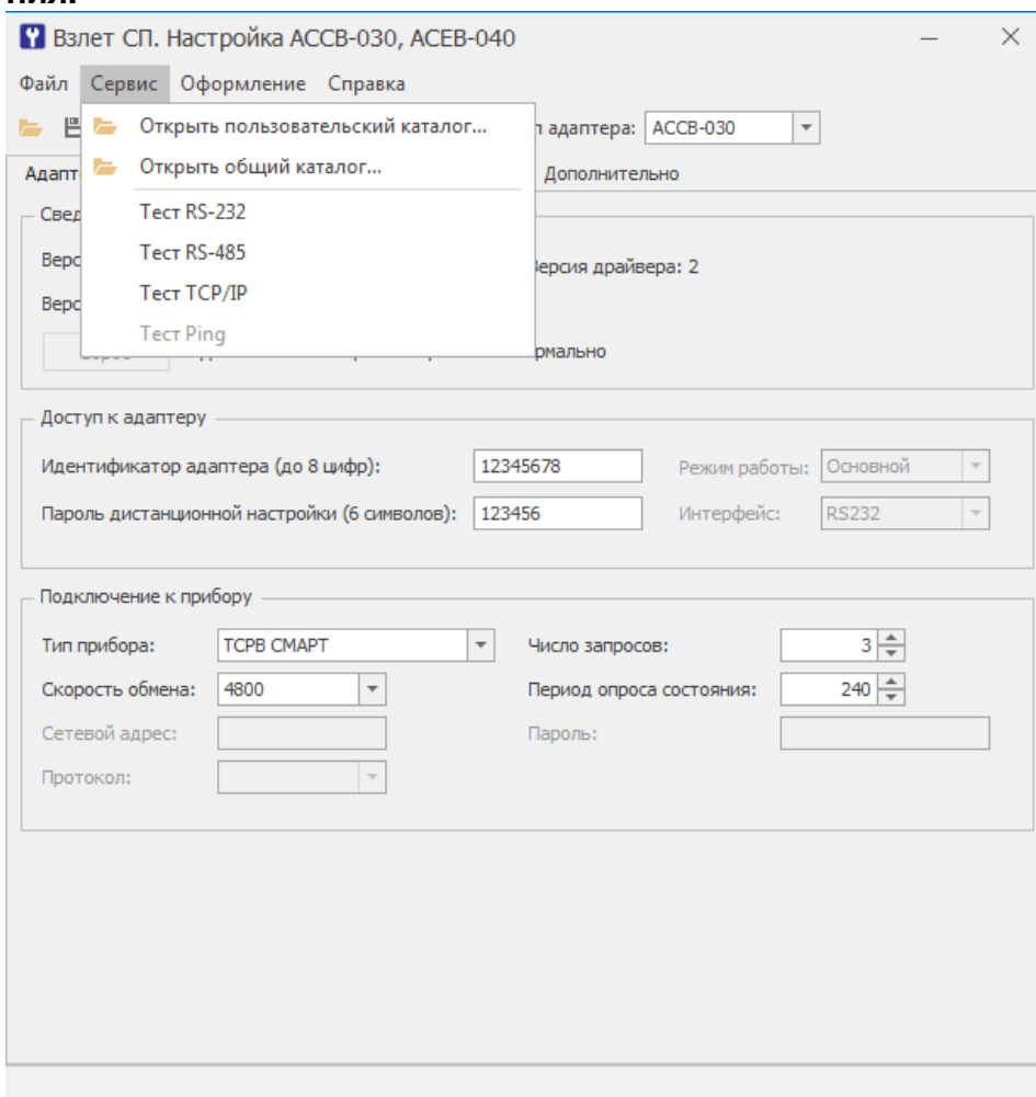
Рис.13. Меню «Сервис» программы «Взлет СП. Настройка АССВ-030, АСЕВ-040».
