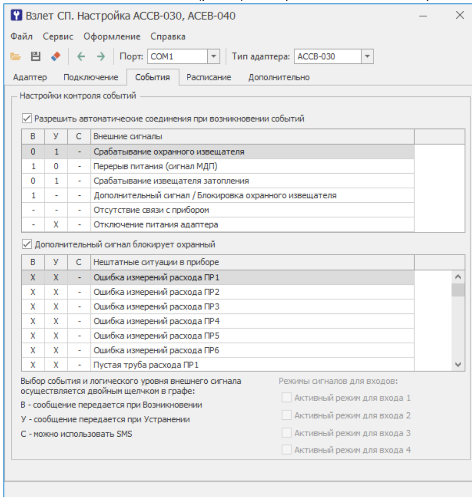
Рис.8. Вкладка «События» программы «Взлет СП. Настройка АССВ-030, АСЕВ-040».
