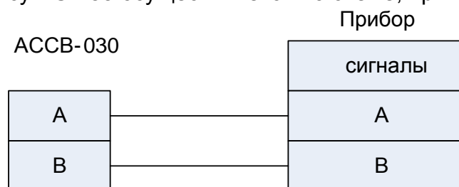
Рис.4. Подключение прибора по интерфейсу RS-485.
