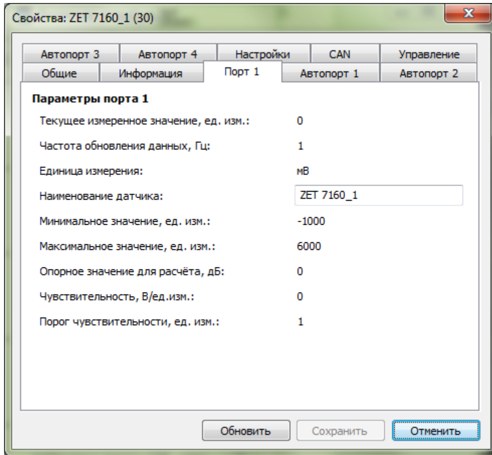
Рис. 4.1 Вкладка «Порт 1»
