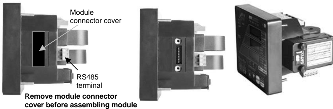
Рисунок 2-36 Типовое подключение
