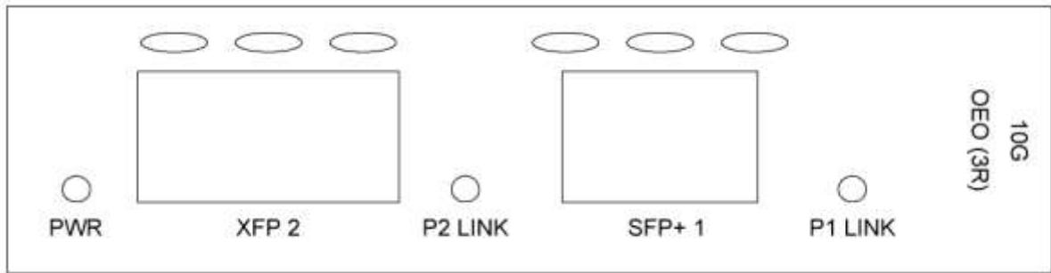
Рисунок 1. Фронтальная панель.
