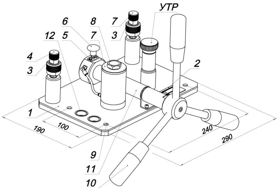
Рисунок 1 – Пресс ПГ-700 с УТР
