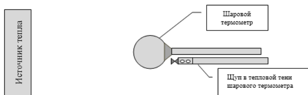
Рис.6 Относительное расположение измерительной аппаратуры и источника излучения.
