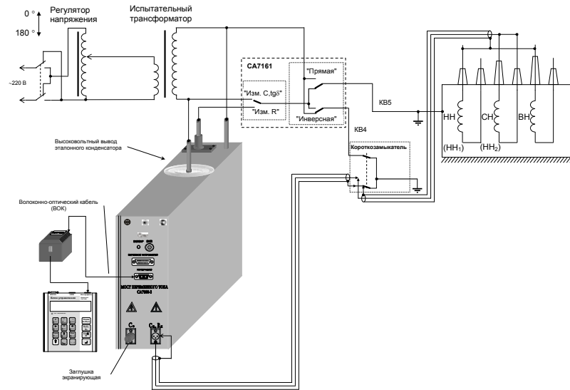
г) СН-бак, "перевернутая (инверсная)" схема
