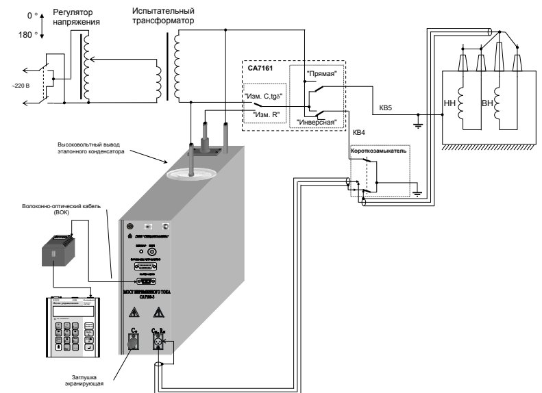
б) (ВН+НН)-бак, "перевернутая (инверсная)" схема
