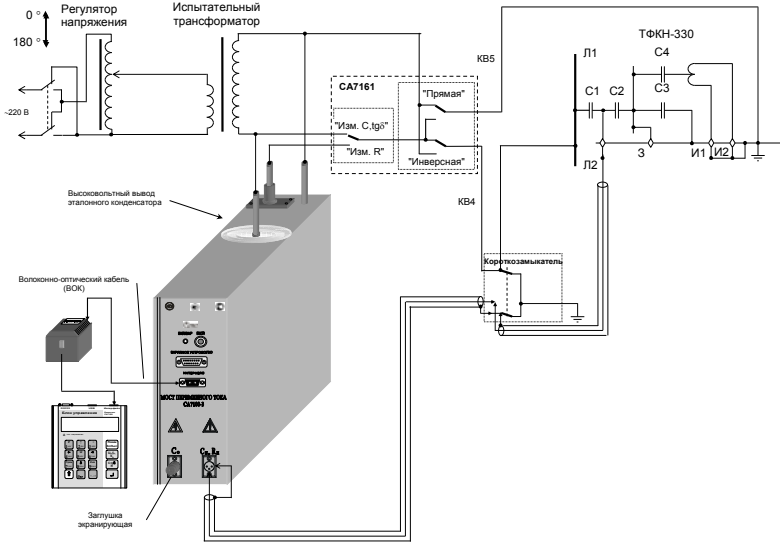
б) измерительного конденсатора, "нормальная (прямая)" схема
