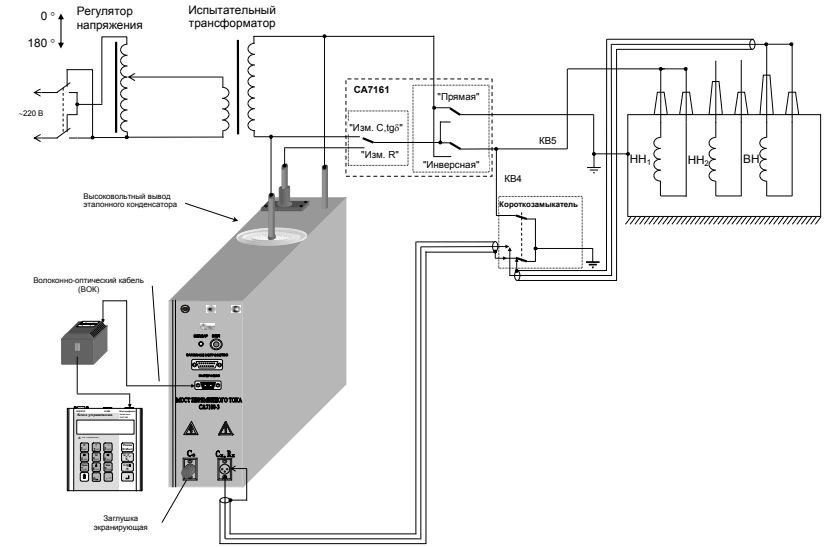
д) ВН-НН1, "нормальная (прямая)" схема
