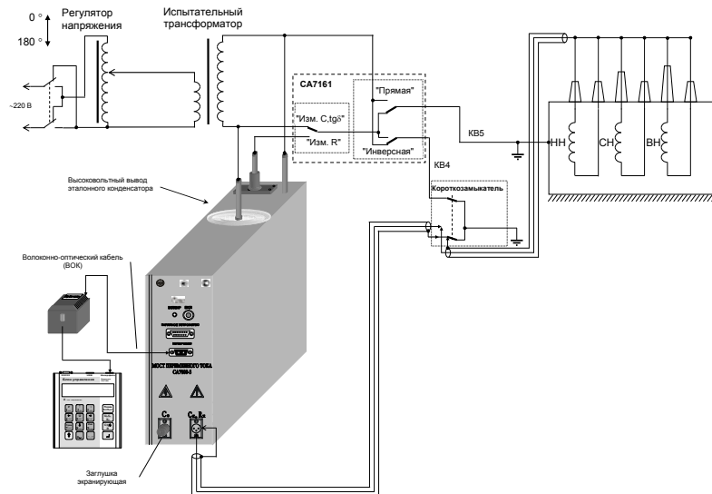
д) (ВН+СН+НН)-бак, "перевернутая (инверсная)" схема.
