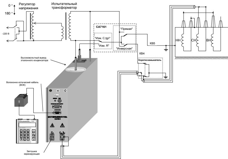
г) СН-бак, "перевернутая (инверсная)" схема
