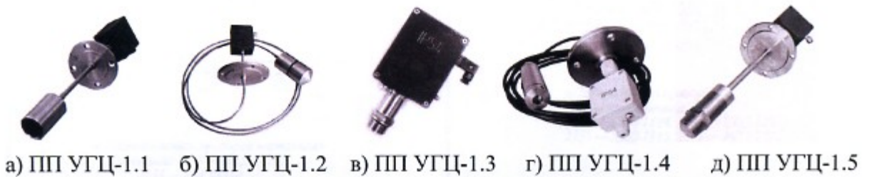
Рисунок 5 – Модель 2170 - передающий преобразователь (ПП) измерителя гидростатического давления цифрового УГЦ-1(-Ex).
