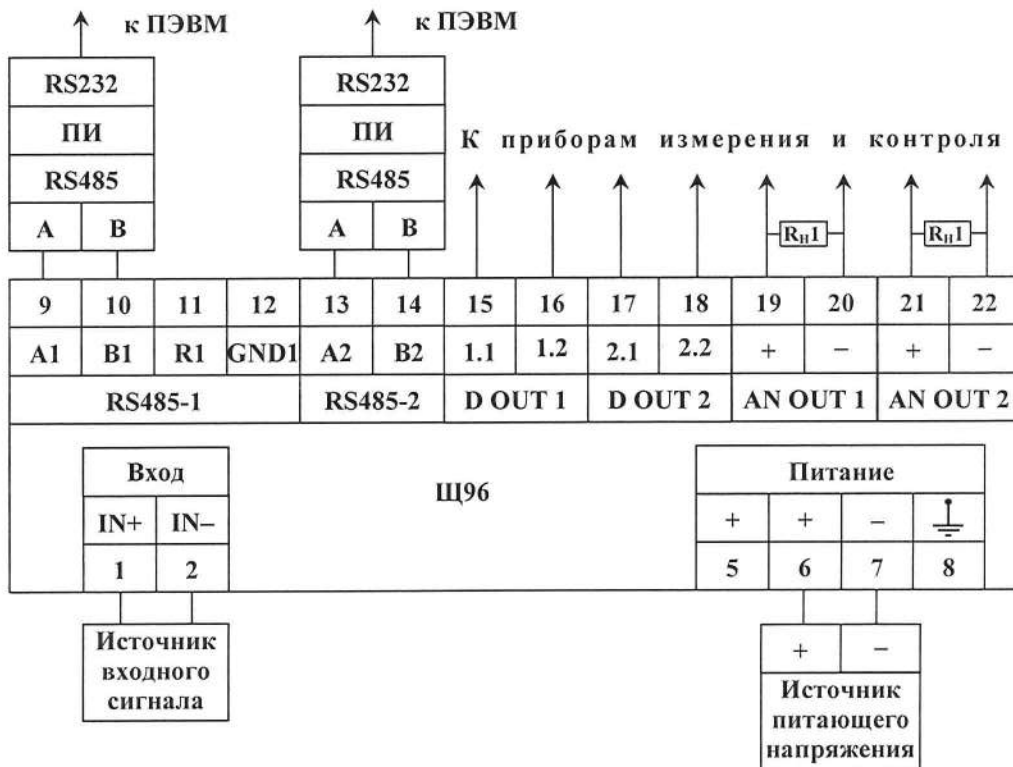
Рисунок Д.2 – Схемы подключения приборов Щ72
