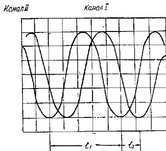
Рис. 8. Измерение разности фаз.
