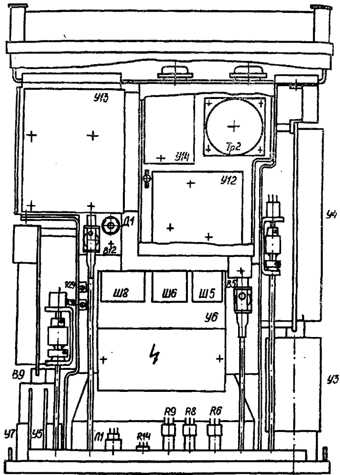
Рис. 6. Вид снизу.
