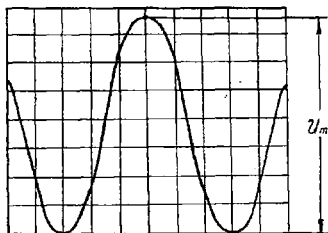
Рис. 3. Измерение полного размаха переменного напряжения.
