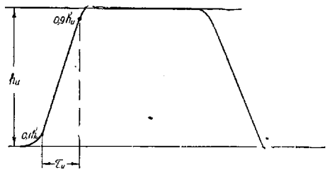
Рис. 12. Измерение времени нарастания.
