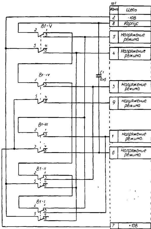
КОММУТАТОР Схема электрическая принципиальная И25.435. 029. Э3
