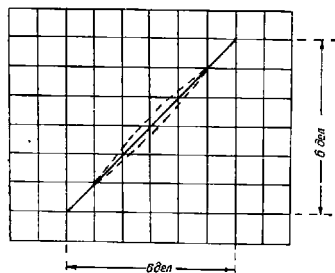
Рис. 14. Форма сигнала в режиме X—Y.
