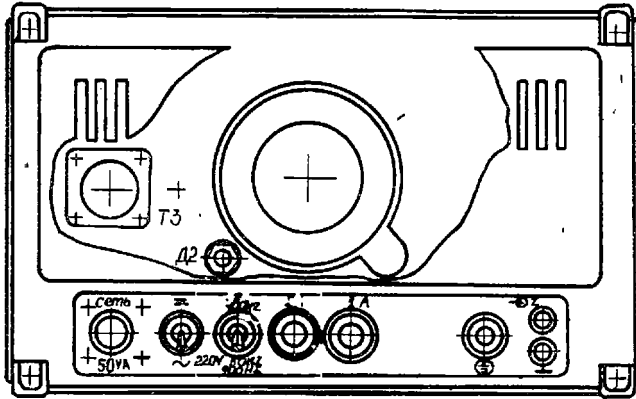
Рис. 4. Вид сзади.
