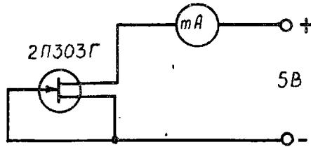
Схема измерения тока стока
