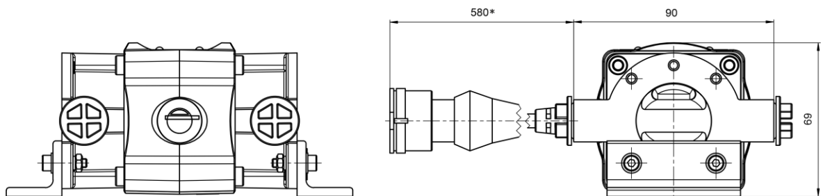
Рисунок А.11 — Габаритные размеры DFM 500S7
