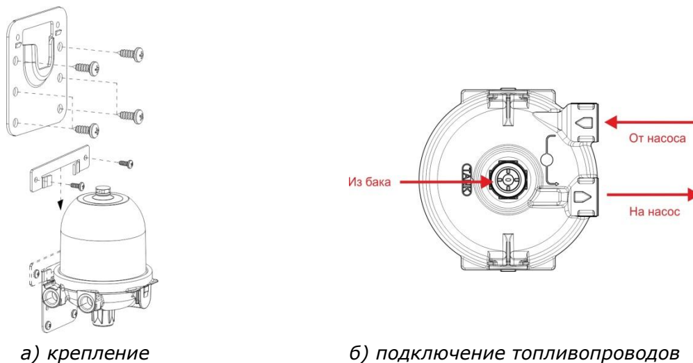
Рисунок 57 — Установка деаэратора DFM DA 250
