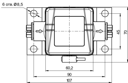
Рисунок А.11 — Габаритные размеры DFM 500S7
