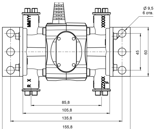
Рисунок А.12 — Габаритные размеры DFM 100DK/D232/D485/DCAN, DFM 100CD и DFM 100DS7
