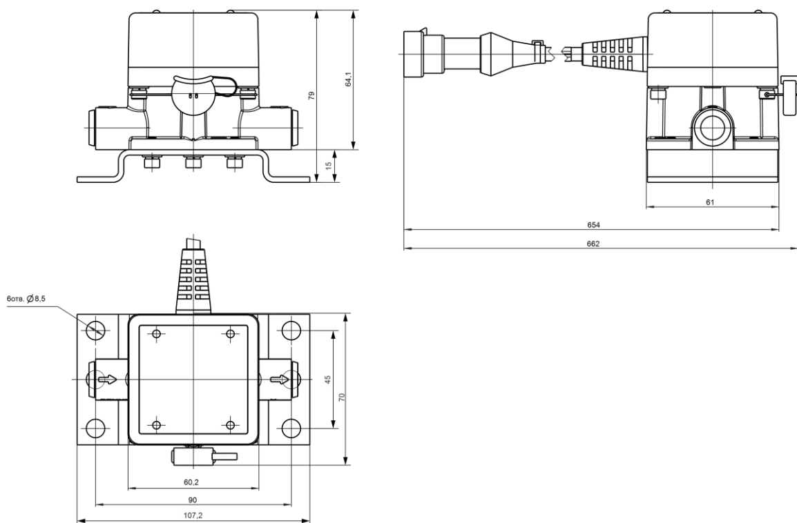
Рисунок А.2 — Габаритные размеры DFM 90AP
