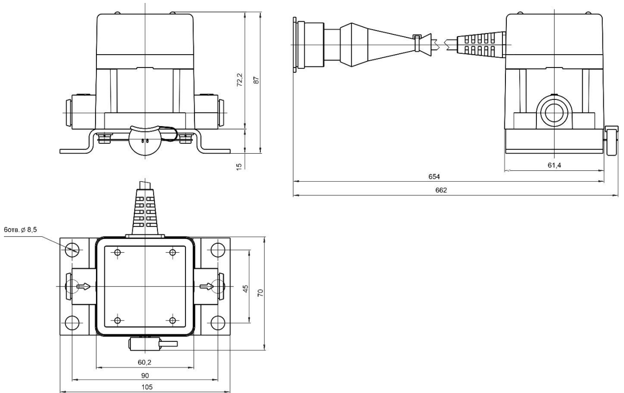
Рисунок А.5 — Габаритные размеры DFM 250AK/CK/A232/A485/ACAN/C232/C485/CCAN
