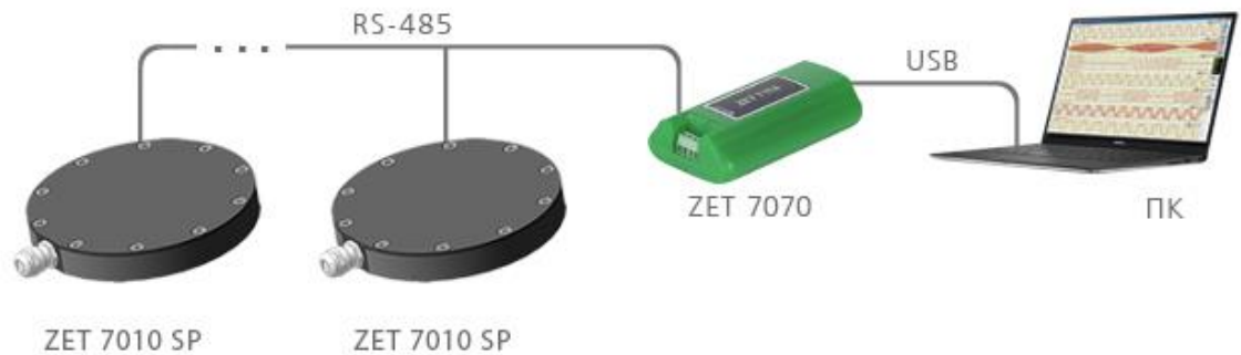
Рис. 2.2 Схема подключения
