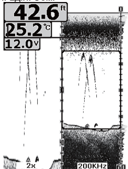
ЭКРАН ЭХОЛОТА С МАСШТАБИРОВАНИЕМ (200 КГц)
