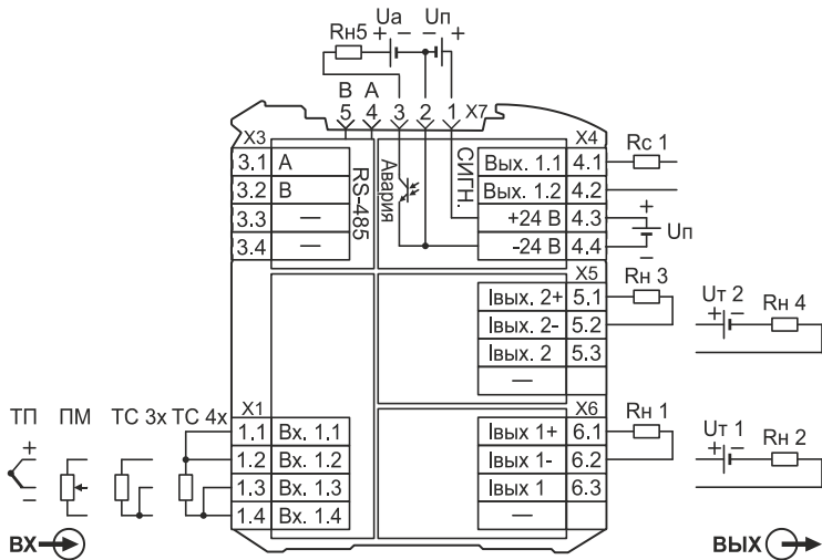
Рисунок 20 – Схема подключения преобразователей НПСИ-250/500-УВ1.2-1С-24-М(22/ЭМР/1Ш/0)
