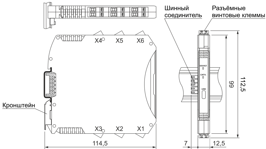
Рисунок 15 – Габаритные размеры преобразователя НПСИ-250/500-УВ1-хС-24-М(12/ТТР/хШ/0)
