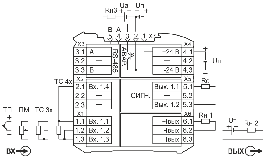
Рисунок 19 – Схема подключения преобразователей НПСИ-250/500-УВ1-хС-24-М(17/ЭМР/хШ/0)
