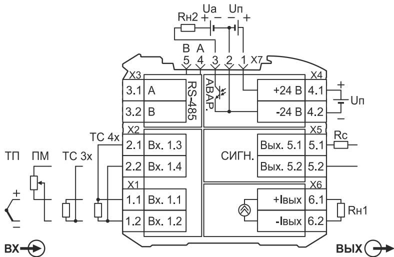
Рисунок 18 – Схема подключения преобразователей НПСИ-250/500-УВ1-хС-24-М(12/ТТР/хШ/0)
