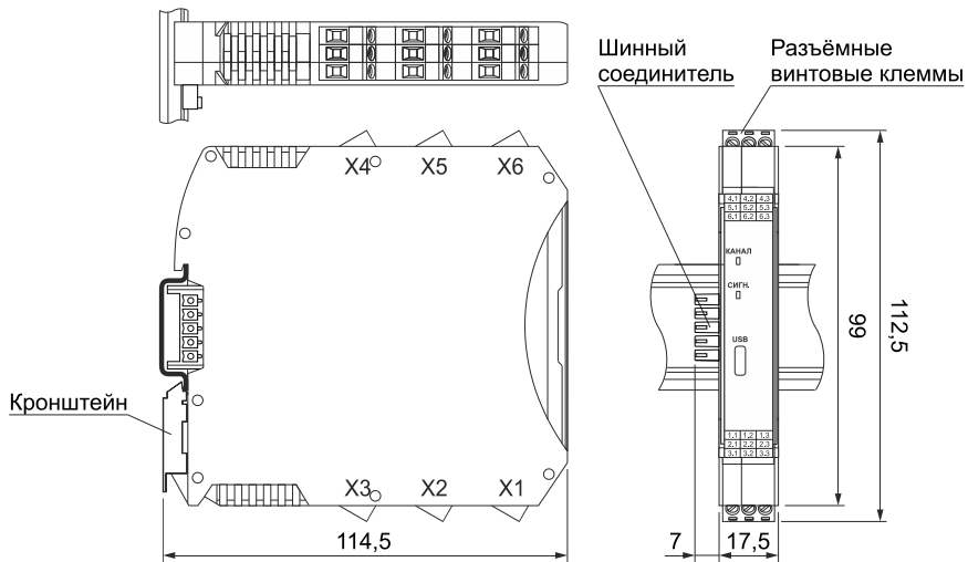
Рисунок 16 – Габаритные размеры преобразователя НПСИ-250/500-УВ1-хС-24-М(17/ЭМР/хШ/0)
