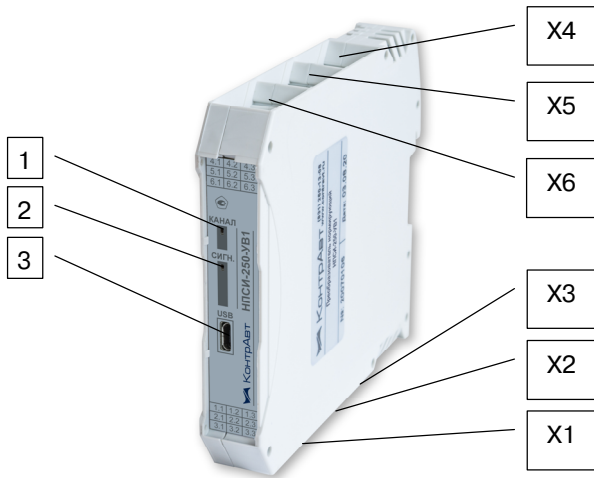
Рисунок 3 – Внешний вид преобразователей НПСИ-250/500-УВ1-хС-24-М(17/ЭМР/xШ/0)
