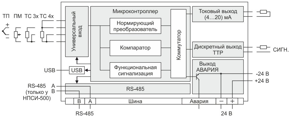
Рисунок 1а – Функциональная структура преобразователей НПСИ-250/500-УВ1-1С-24-М(12/ТТР/1Ш/0)
