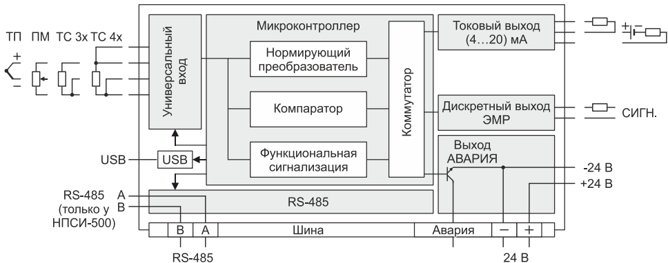
Рисунок 16 – Функциональная структура преобразователей НПСИ-250/500-УВ1-1С-24-М(17/ЭМР/1Ш/0)
