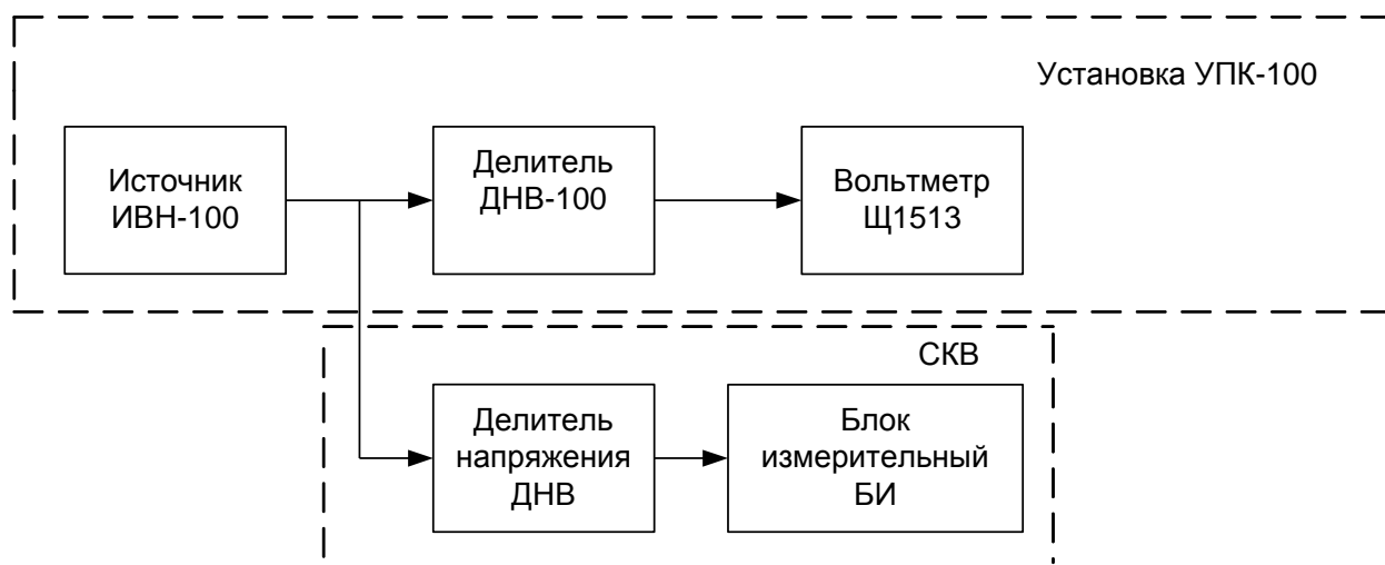
Рисунок 5 – Схема подключение СКВ к УПК-100
