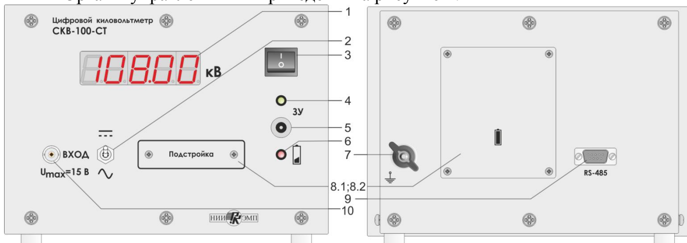
а) – Внешний вид передней панели стационарного БИ
