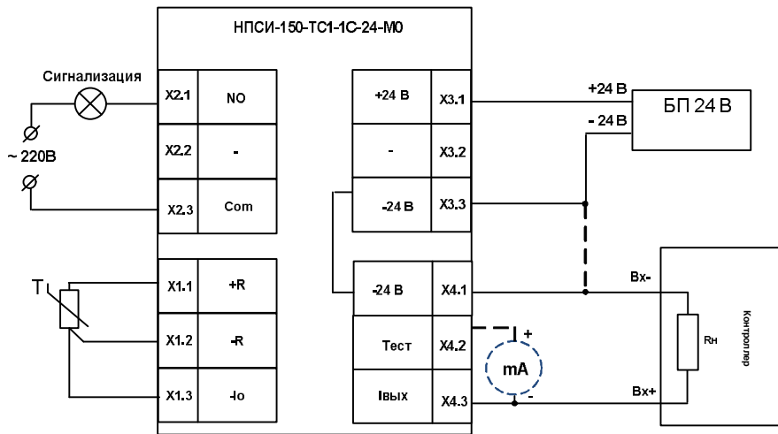
Рисунок 9 – Схема подключения преобразователей НПСИ-150-ТС1-1С-24-М0
