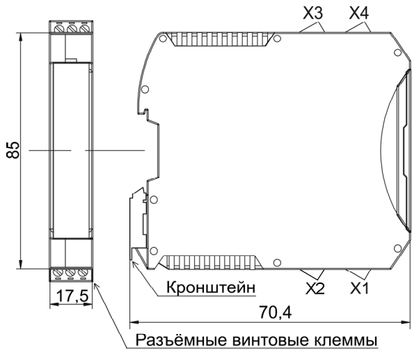
Рисунок 8 – Габаритные размеры преобразователя
