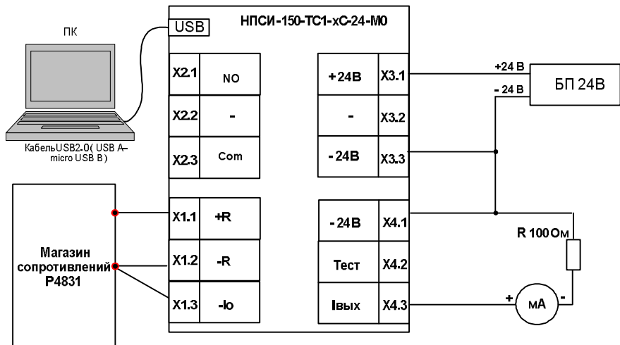
Рисунок А.6.4.1 – Подключение преобразователей НПСИ-150-ТС1 для проведения поверки преобразования сопротивления в выходной токовый сигнал от 4 до 20 мА
