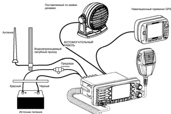
Рис. 1. Общая установка
