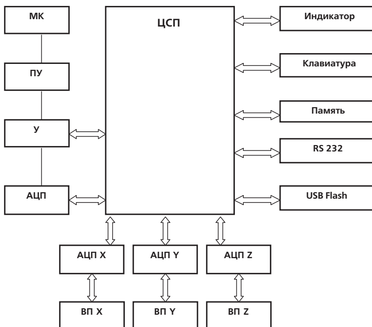
Рис. 2.2. Функциональная схема прибора.
