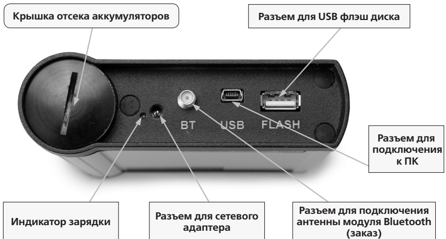
Рисунок 2.1.2. Нижний фланец прибора
