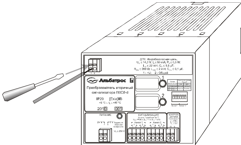
Рисунок 3 – Подключение электрических цепей к прибору
