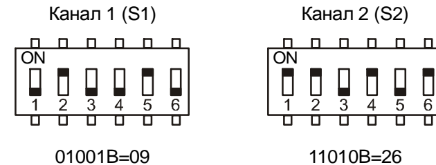
Рисунок 7 – Положение секций переключателей для рассматриваемого примера
