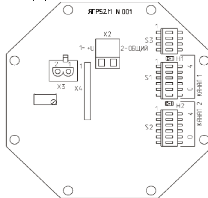
Рисунок 5 – Расположение переключателей задания уставок и светодиодов на плате ЯПР52М
