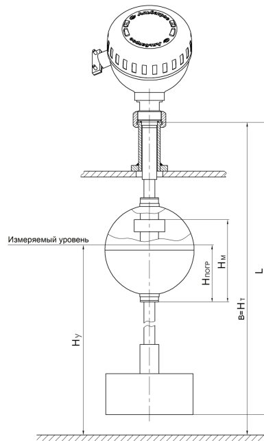
Рисунок 6 – Схема определения уровня срабатывания прибора
