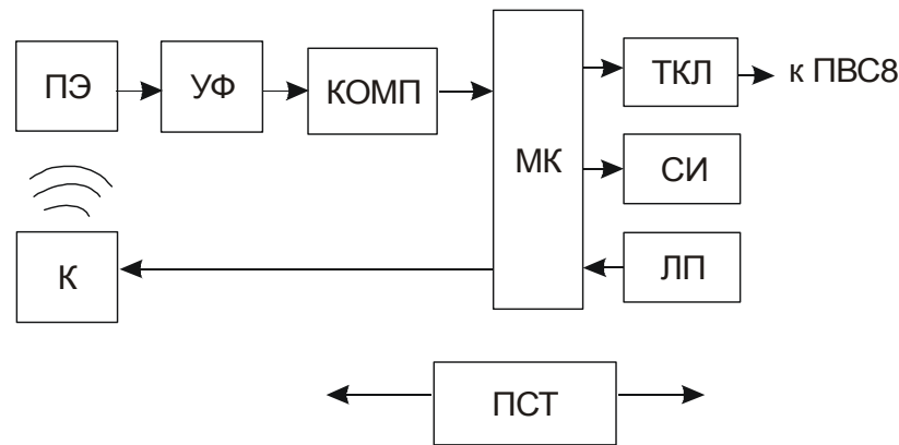
Рисунок 1 – Структурная схема датчиков
