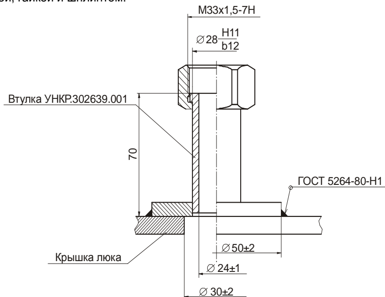
Рисунок 2 – Рекомендуемое посадочное место для установки датчика
