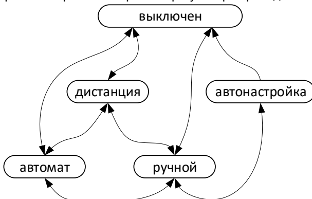
Рисунок 2.7. Управление ПИД-регулятором
