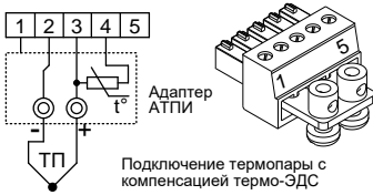
Рисунок Б.1 – Подключение датчиков к каналам АВ.
