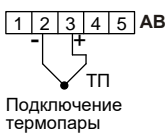
Рисунок Б.1 – Подключение датчиков к каналам АВ.
