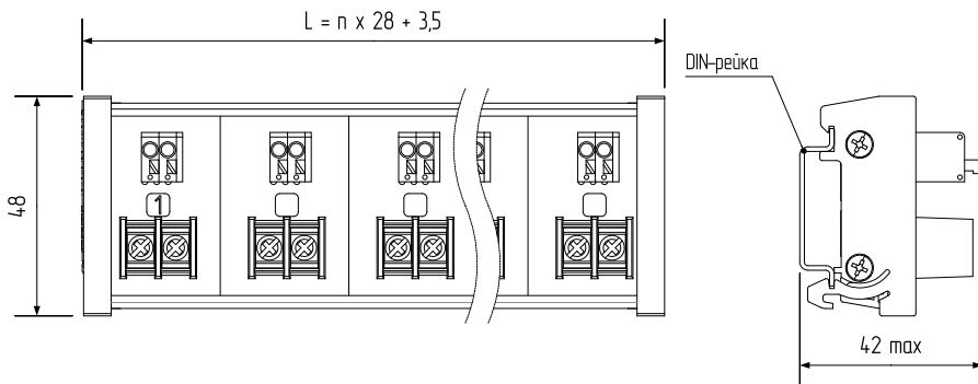
Рисунок Б.10 Адаптер nАДЧ (ДВ-ЧВ). Габаритные и установочные размеры n = 1...8 – кол-во каналов в одном держателе на DIN-рейку
