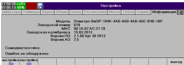
Рисунок 2.34 Меню «Информация»
