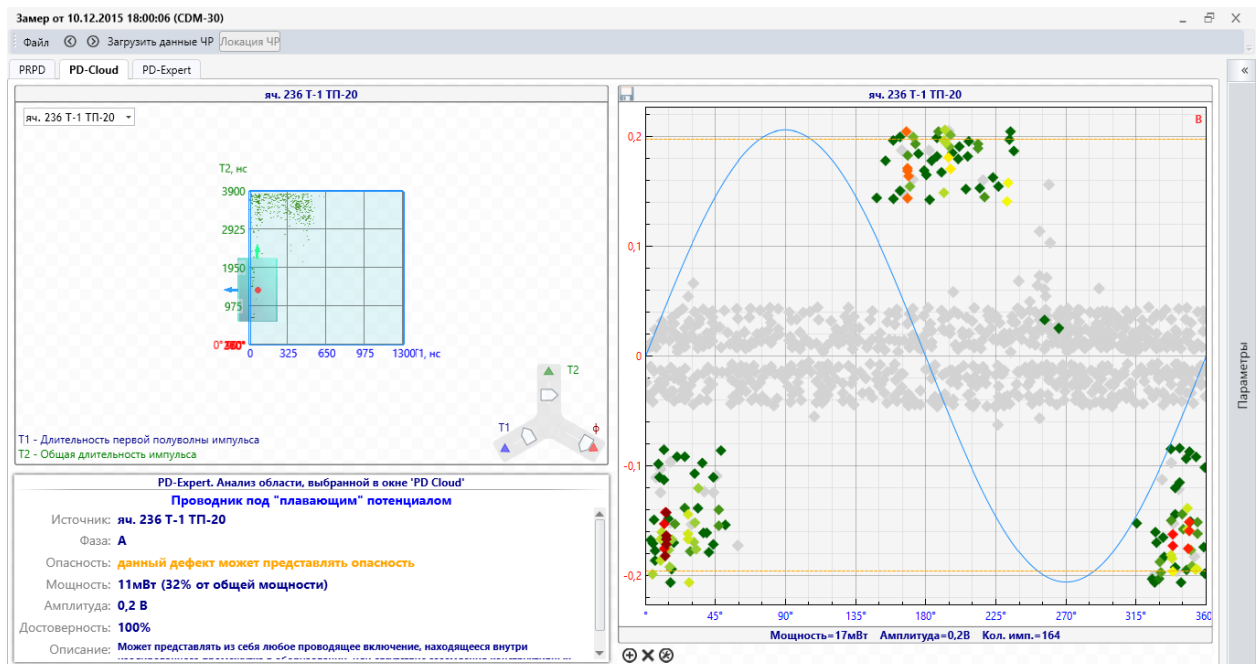
Рисунок 40 Окно TPI-распределения
