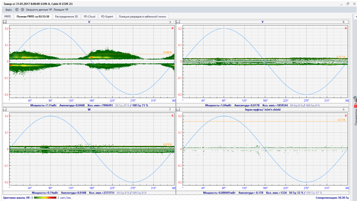
Рисунок 38 Полная PRPD
