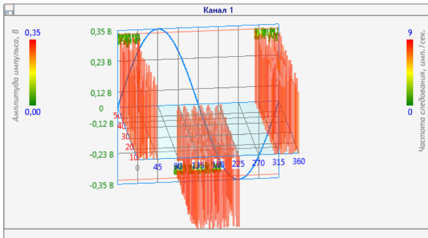
Рисунок 39 3d распределение
