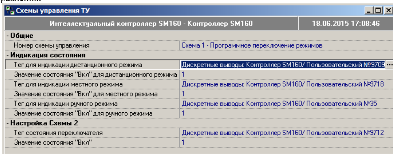
Рисунок 30– Схемы управления ТУ
