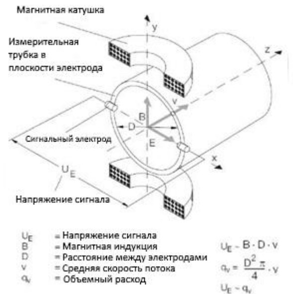
Схема электромагнитного расходомера
