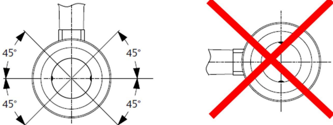
Рисунок 12 - Расположение электродов
