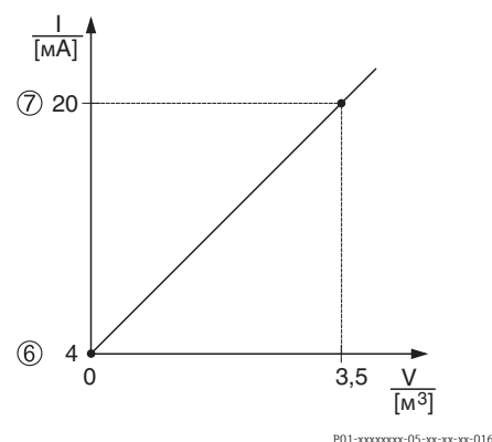
Рис. 16: Ручной ввод таблицы линейаризации
