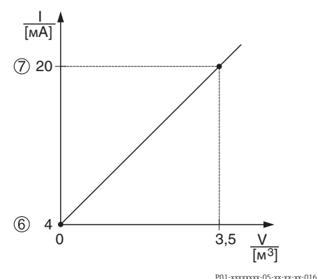
Рис. 15: Полуавтоматический ввод таблицы линейризации
