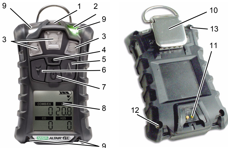
Рис. 1 Обзор прибора
