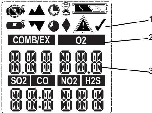
Рис. 2 Дисплей
