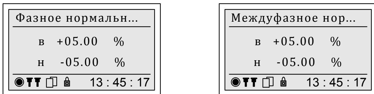
Рисунок 54 – Отображение нормально допустимых значений отклонений фазного и междуфазного напряжения для отклонения среднеквадратического значения напряжения и отклонения напряжения основной частоты
