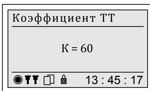
Рисунок 50 – Меню «Коэффициент ТТ»
