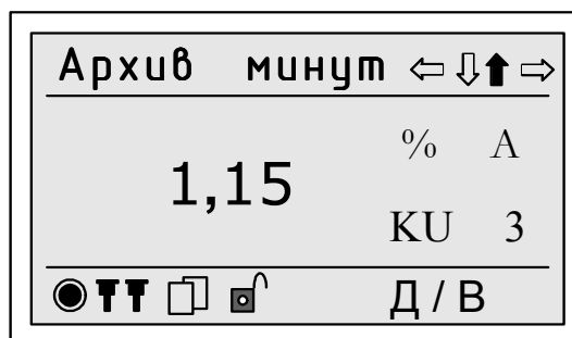
Рисунок 11 – Пример отображения на дисплее счетчика результатов измерений ПКЭ на объединённом интервале времени 1 мин
