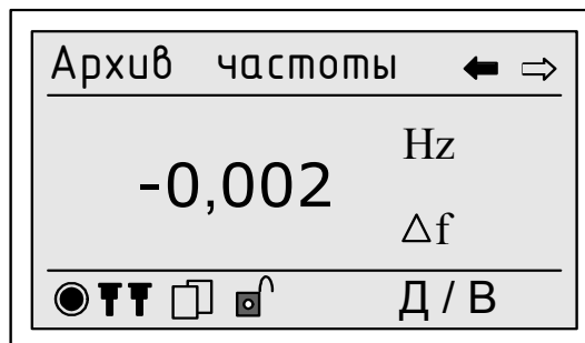
Рисунок 9 – Пример отображения на дисплее счетчика результатов измерений отклонения частоты
