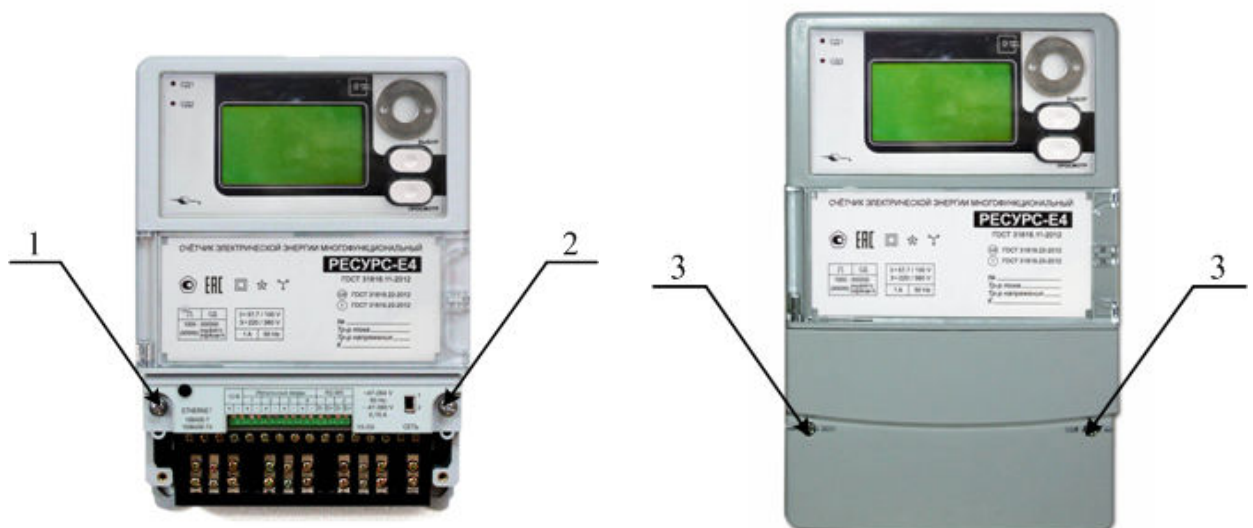
Рисунок А.1 – Внешний вид и схема пломбирования модификаций счетчика «Ресурс-Е4-Х-Х-В-Х»
