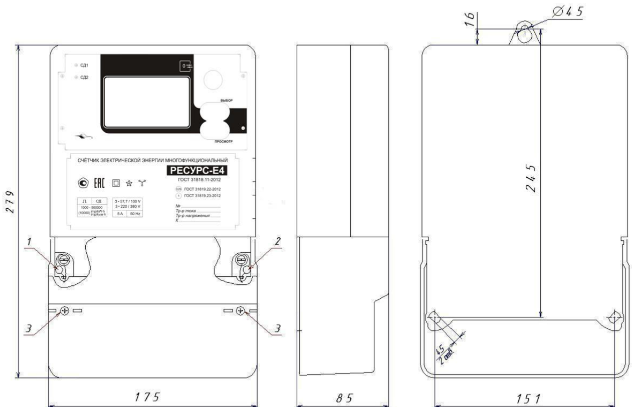
Рисунок А.3 – Габаритные размеры модификаций счетчика «Ресурс-Е4-Х-Х-В-Х»
