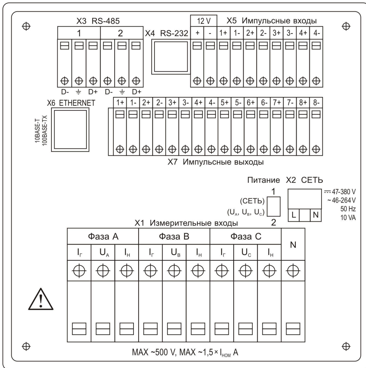
Рисунок Б.1 – Разъёмы модификаций счетчика «Ресурс-Е4-Х-Х-В-Х»
