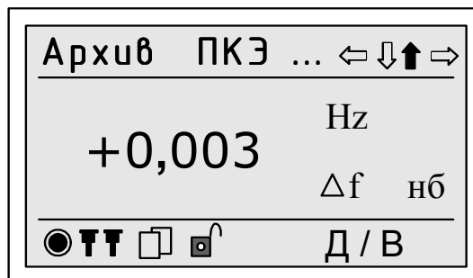
Рисунок 14 – Пример отображения на дисплее счетчика значений статистических характеристик ПКЭ за одни сутки
