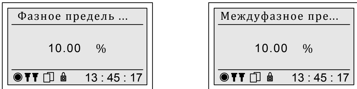
Рисунок 57 – Отображение предельно допустимых значений отклонений фазного и междуфазного напряжения для положительного и отрицательного отклонений напряжения
