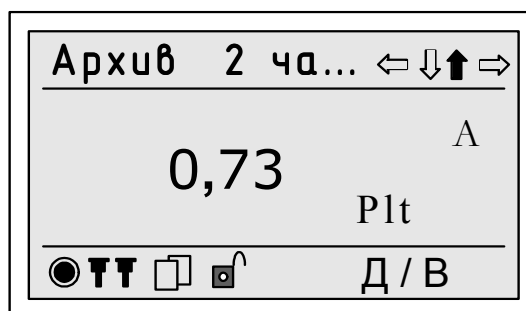
Рисунок 13 – Пример отображения на дисплее счетчика результатов измерений ПКЭ на объединённом интервале времени 2 ч
