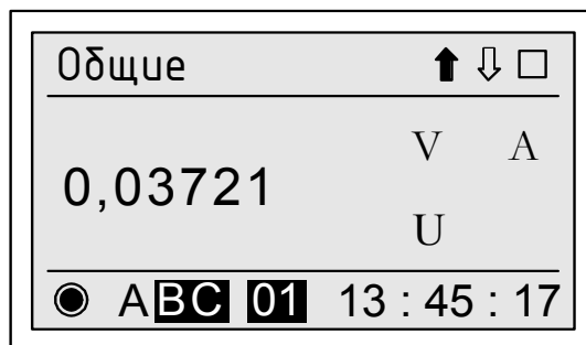
Рисунок 5а – Пример отображения сообщения об отсутствии фазного напряжения
