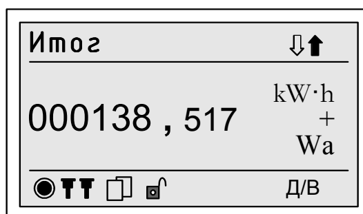
Рисунок 18 - Пример вывода результатов измерений активной энергии за все время работы счетчика с момента пуска
