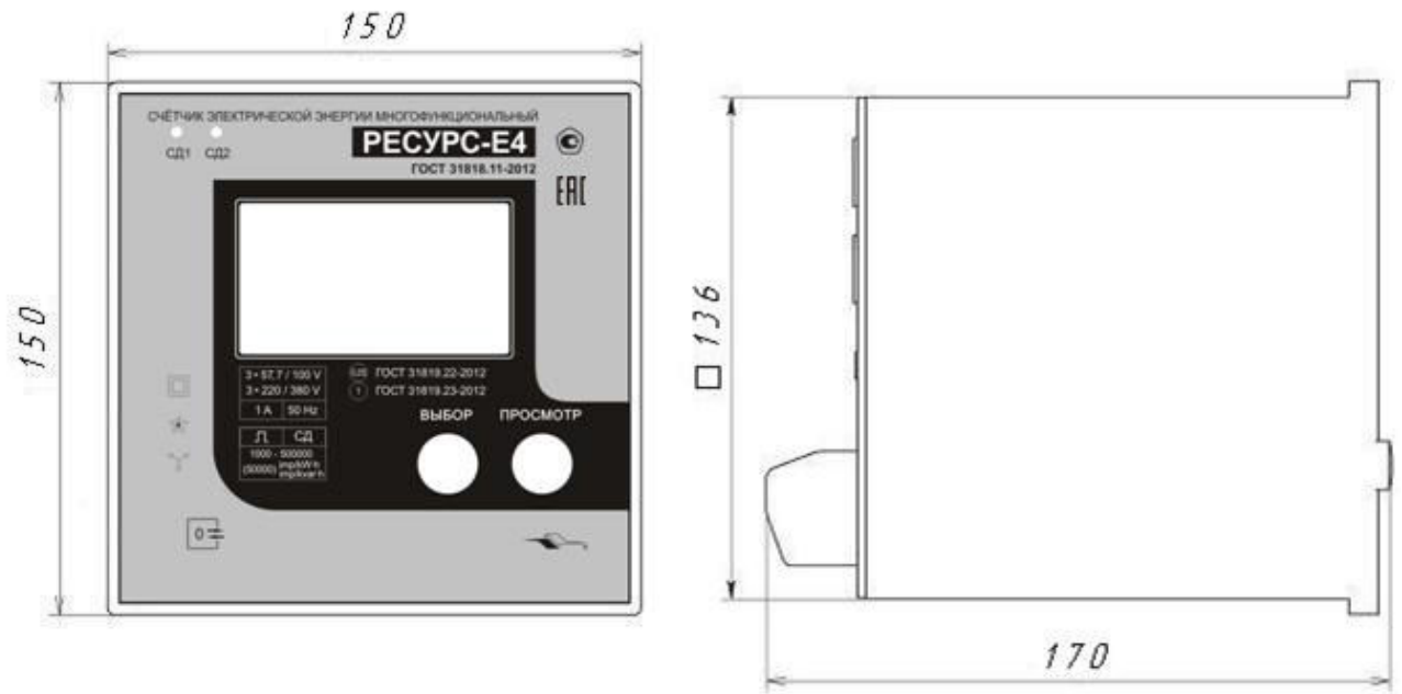
Рисунок А.3 – Габаритные размеры модификаций счетчика «Ресурс-Е4-Х-Х-В-Х»
