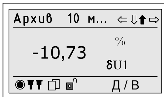
Рисунок 12 – Пример отображения на дисплее счетчика результатов измерений ПКЭ на объединённом интервале времени 10 мин
