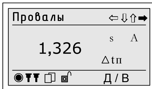
Рисунок 16 – Пример отображения на дисплее счетчика результата измерения длительности провала напряжения
